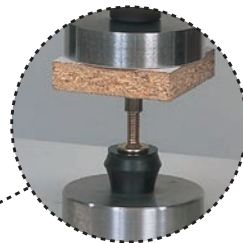
支持脚単体強度試験
