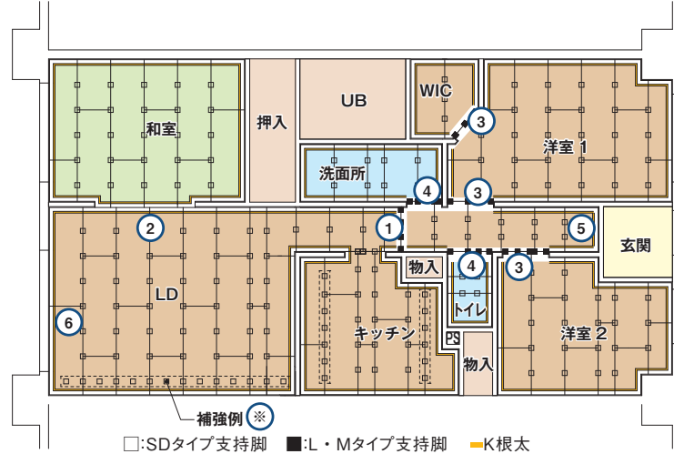
□:SDタイプ支持脚 ■:L・Mタイプ支持脚 ●:K根太
