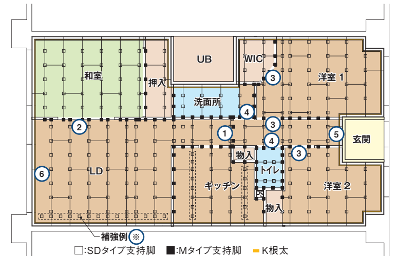
□:SDタイプ支持脚 ■:Mタイプ支持脚 ●:K根太
