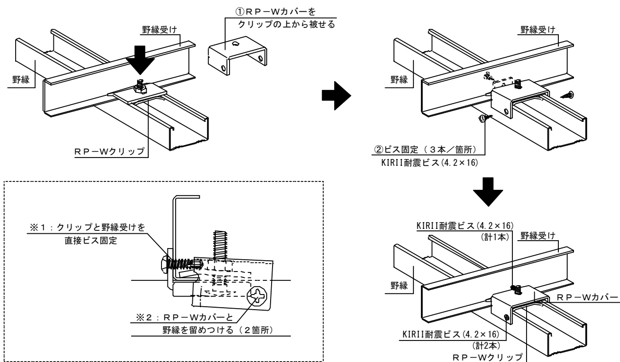
図 2-5-13 RP-Wカバー施工方法
