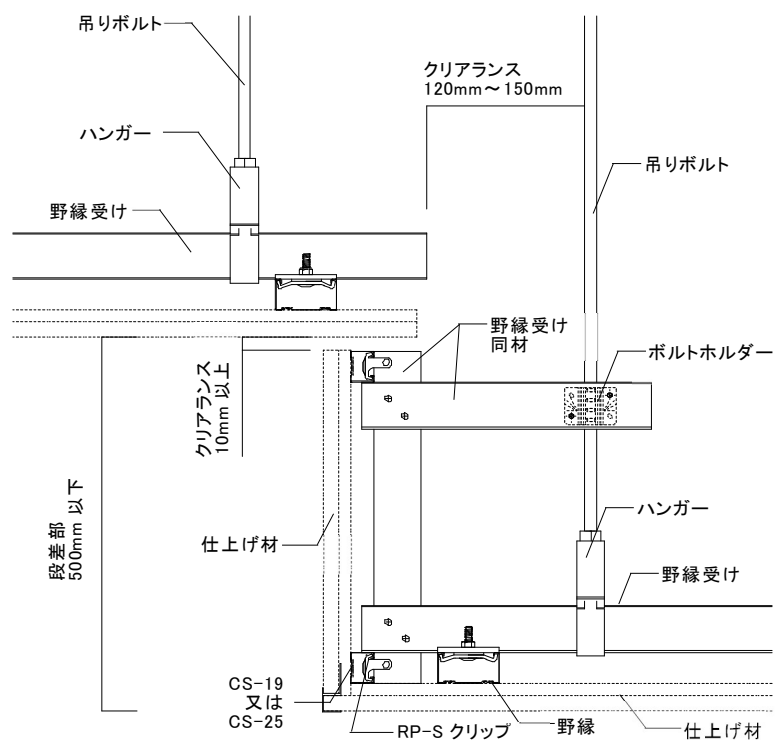
中間折上げ(直角)の場合 図 3-2-1 (参考例)段差部クリアランス
