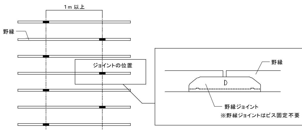
図 2-4-3 野縁の継手
