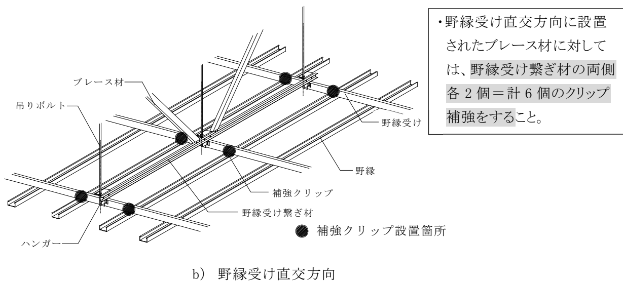
図 2-5-14 補強クリップ設置箇所
