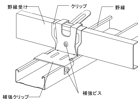
図 2-4-1 補強部のクリップ
