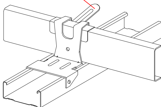
a) 補強クリップ(背掛け)
