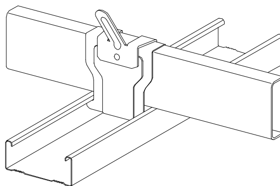
b) 補強クリップ(腹掛け)
