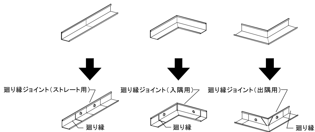
b)廻り縁ジョイント(ビス)の場合
