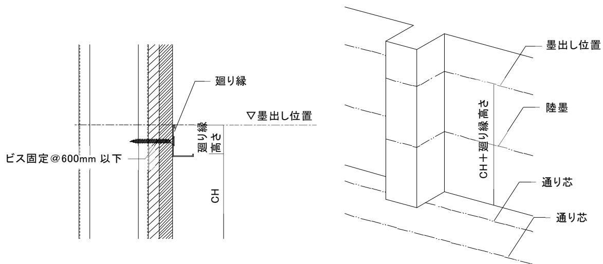
図2-1-1 墨出し位置
