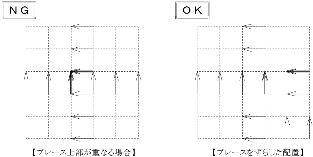
図2-7-10 ブレースの配置例①
