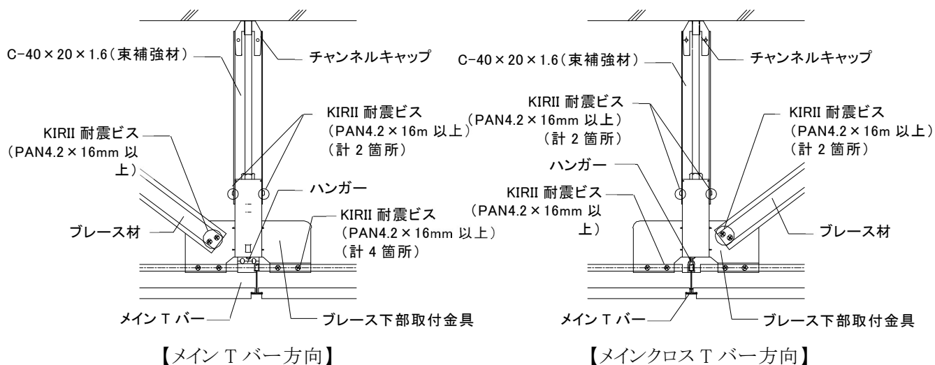
図 1-2-2 ブレース設置部の名称
