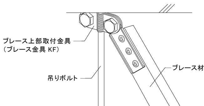
図 2-7-4 ブレース上部取付詳細②
