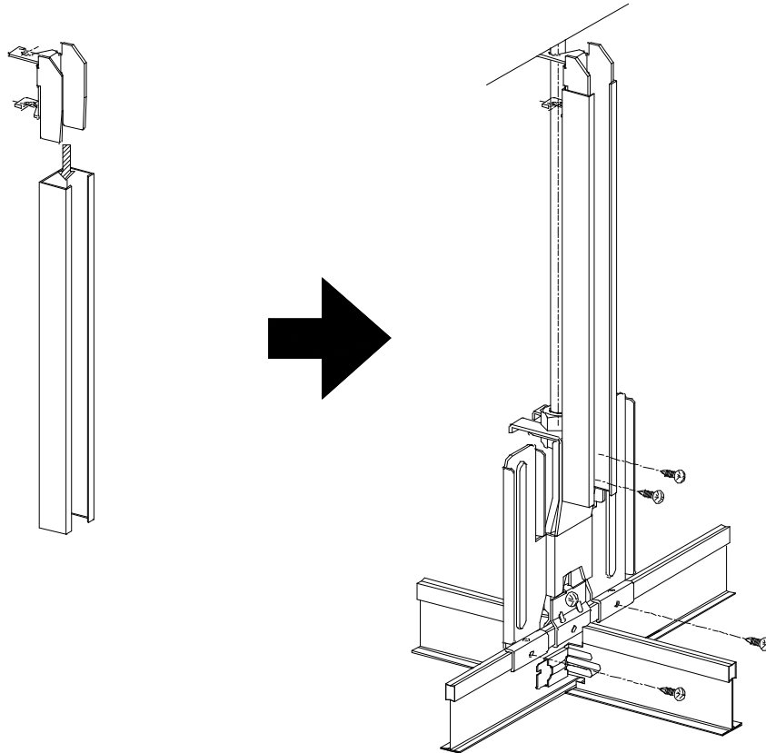
図2-7-10 束補強材取付詳細
