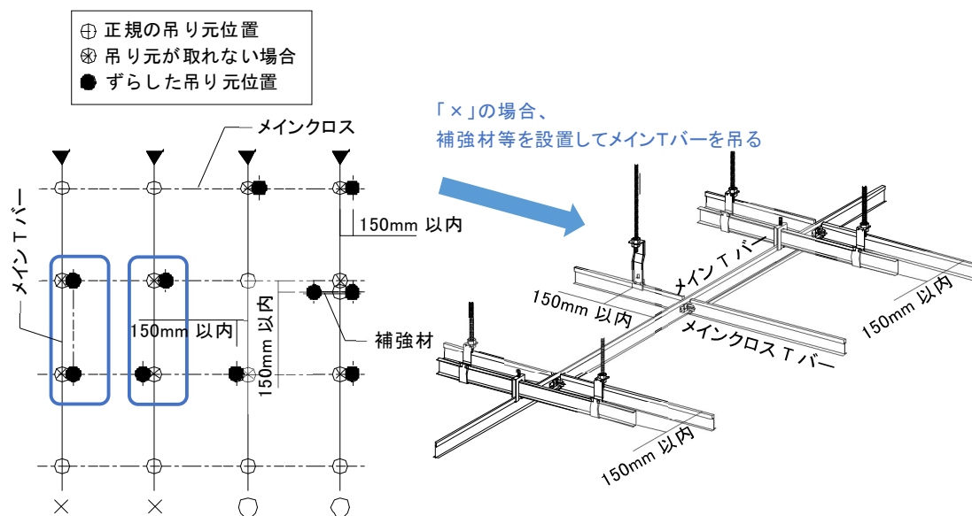
図2-3-3 吊りボルト設置時の注意事項
