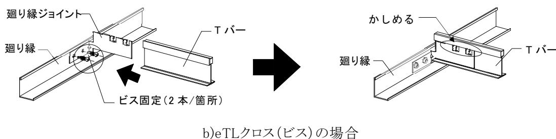
図2-4-5 Tバーと廻り縁の接続
