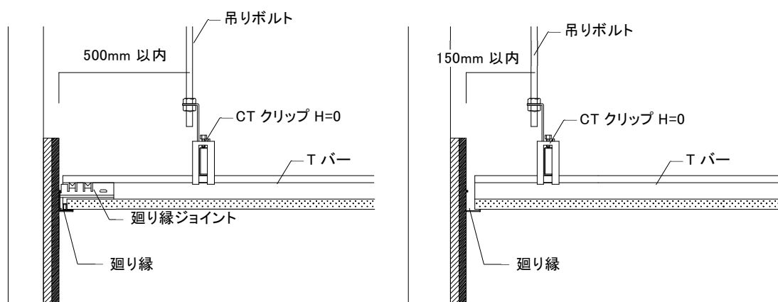
a) 廻り縁ジョイントを施工する場合
