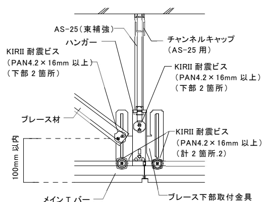
【メイン T バー方向】
