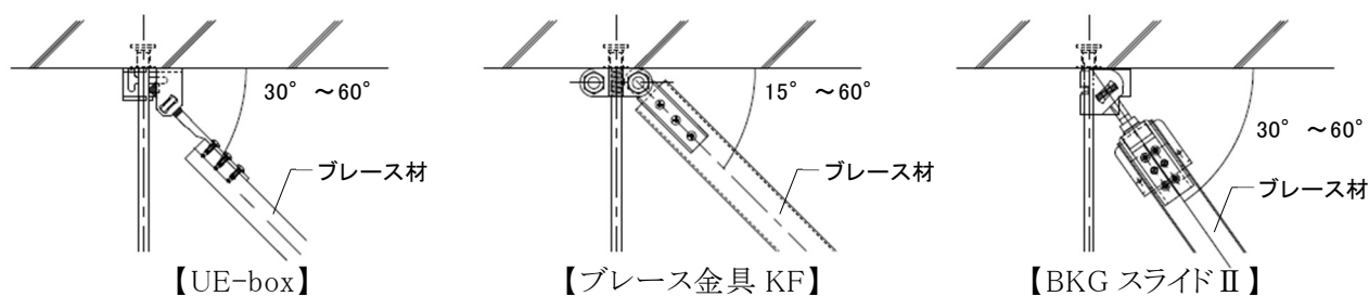
図 2-7-8 ブレース設置角度
