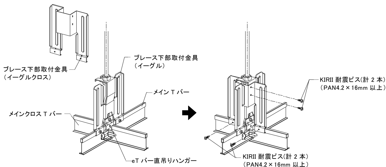
図2-7-2 ブレース下部取付金具(イーグルクロス)の設置
