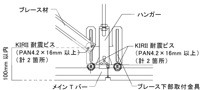
【メイン T バー方向】
