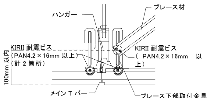
【メインクロス T バー方向】
