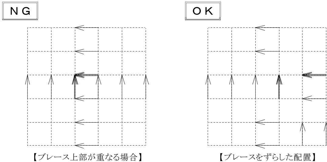
図2-7-11 ブレースの配置例①
