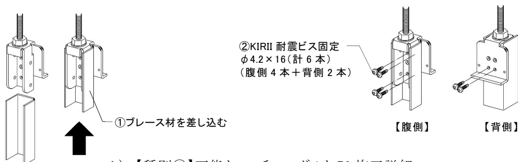
b) 【種別④】万能キャッチャーボルト 70 施工詳細
