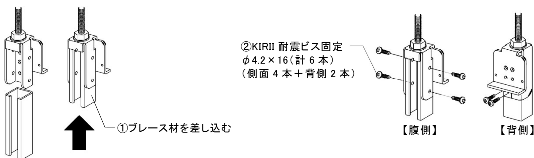
a) 【種別③】万能キャッチャーボルト 70 の施工方法
