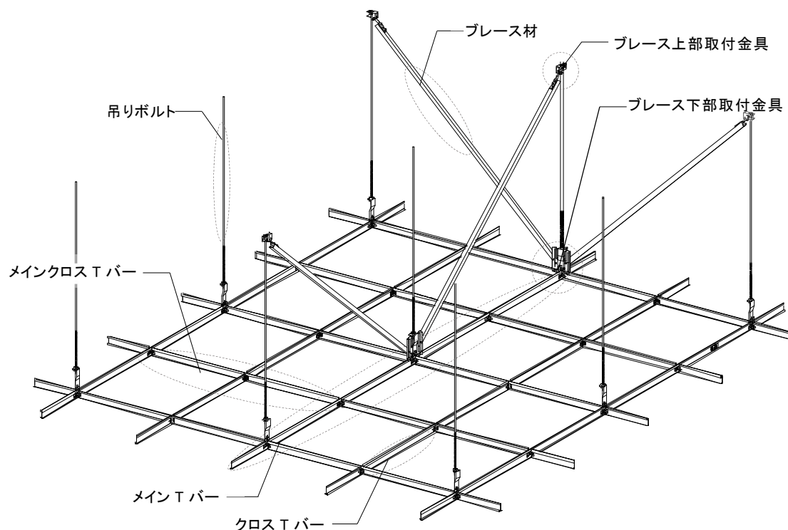
図 1-2-1 各部の名称(例図)
