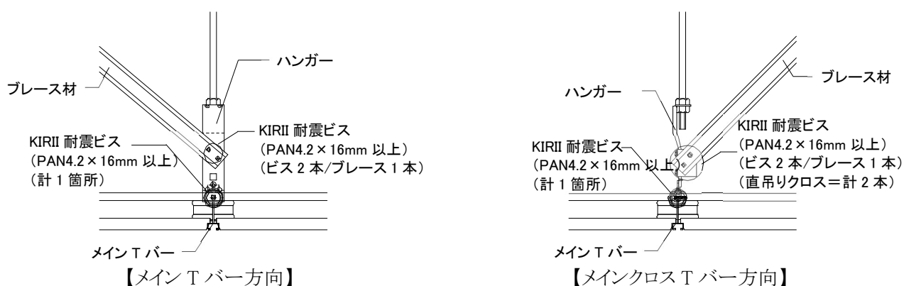
図2-7-7 ブレース下部取付詳細
