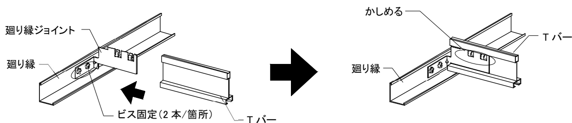
b)eTLクロス(ビス)の場合
