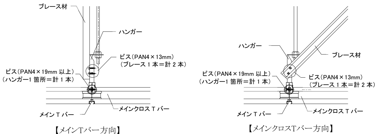
図2-7-7 ブレース下部取付詳細
