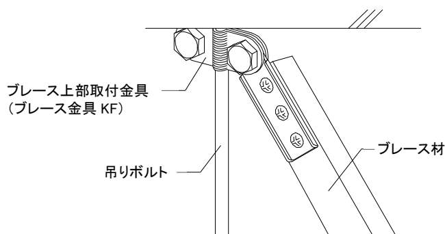
図 2-7-2 ブレース上部取付け詳細②
