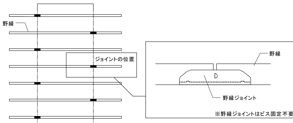
図 2-4-2 野縁の継手
