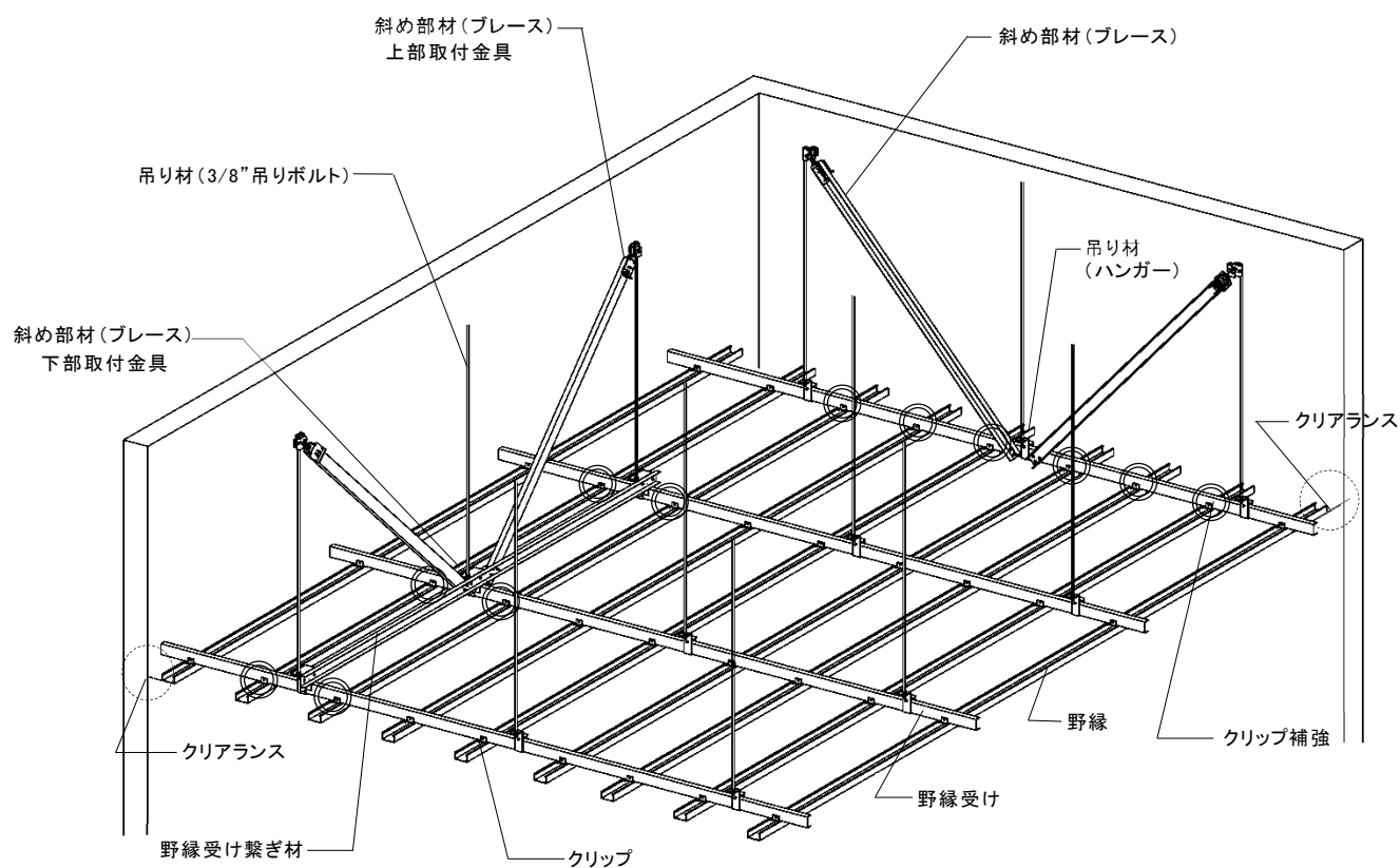
図 1-2-1 耐震 FullPower 天井(強化)(例図)
