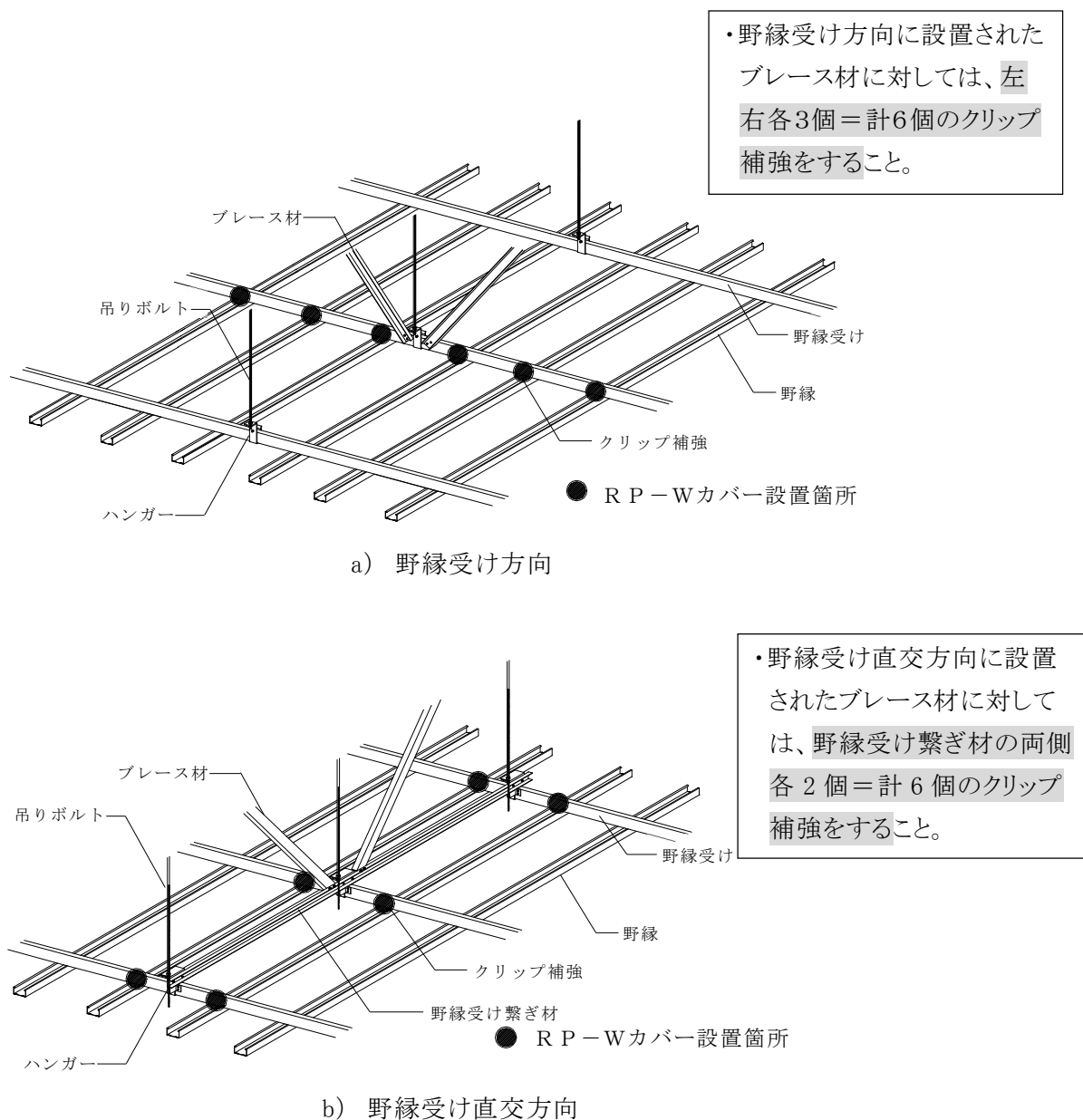
図 2-5-13 クリップ補強の施工箇所
