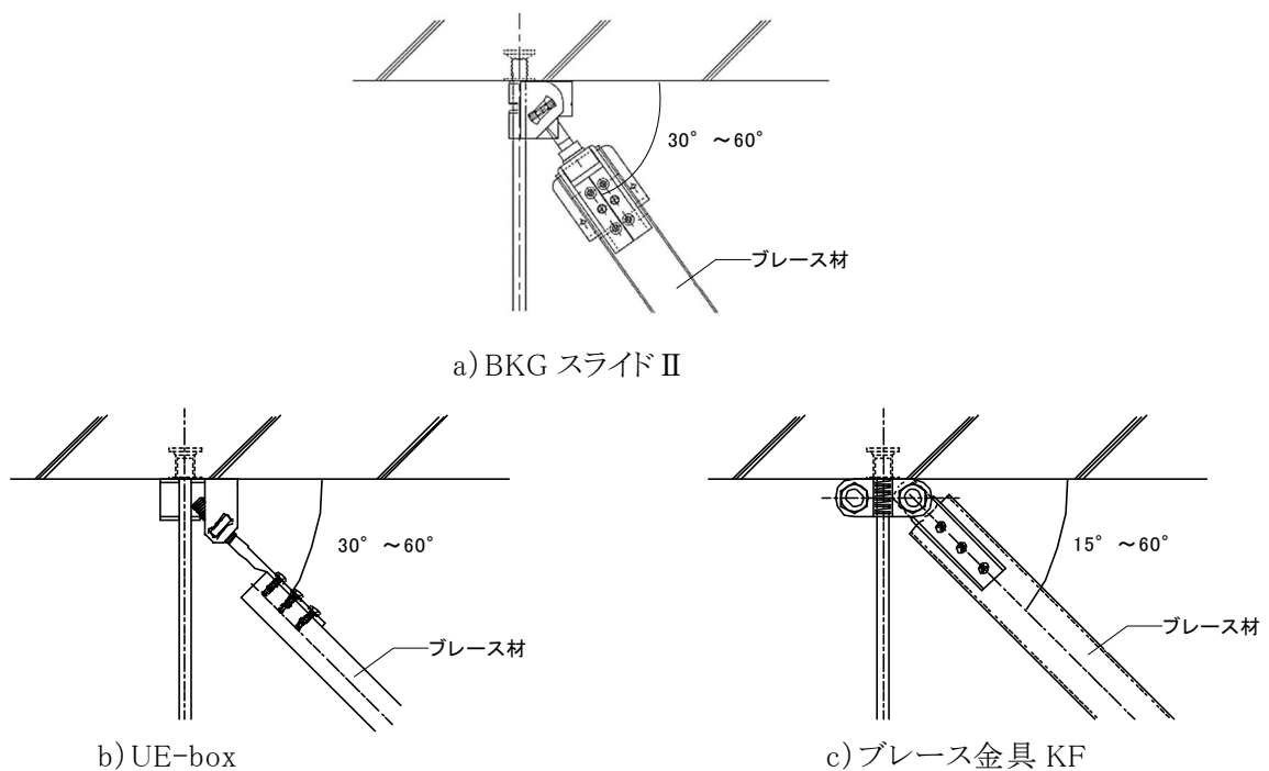
図 2-5-8 ブレース設置角度
