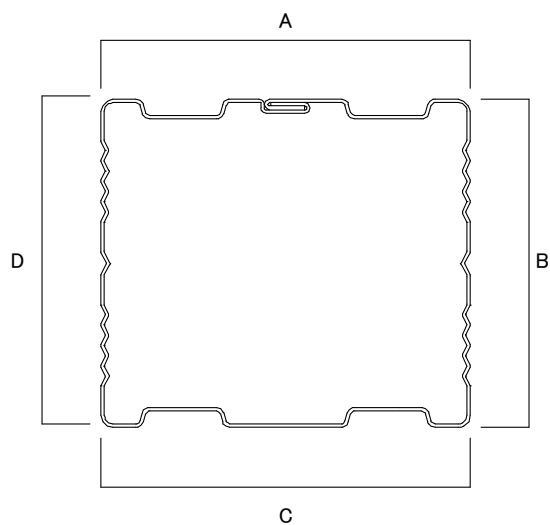
図 1-4-1 SQ-BAR 断面図
