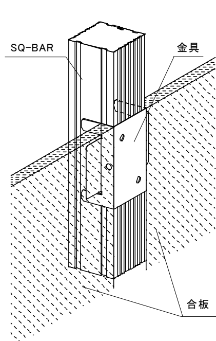
図 2-7-2 (参考) 合板による補強
