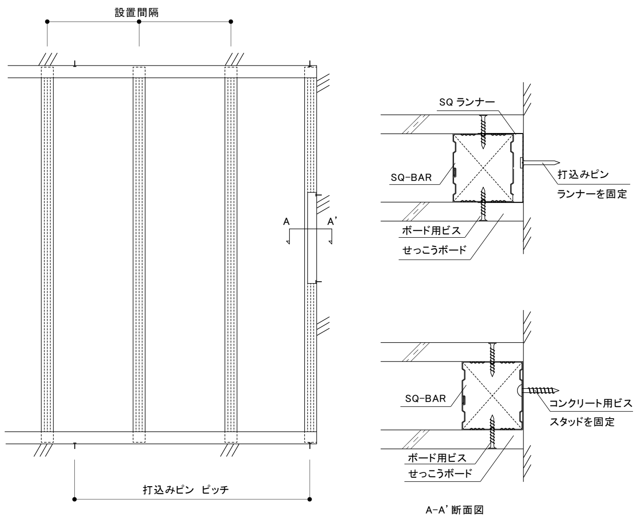
図 2-4-1 壁端部の施工
