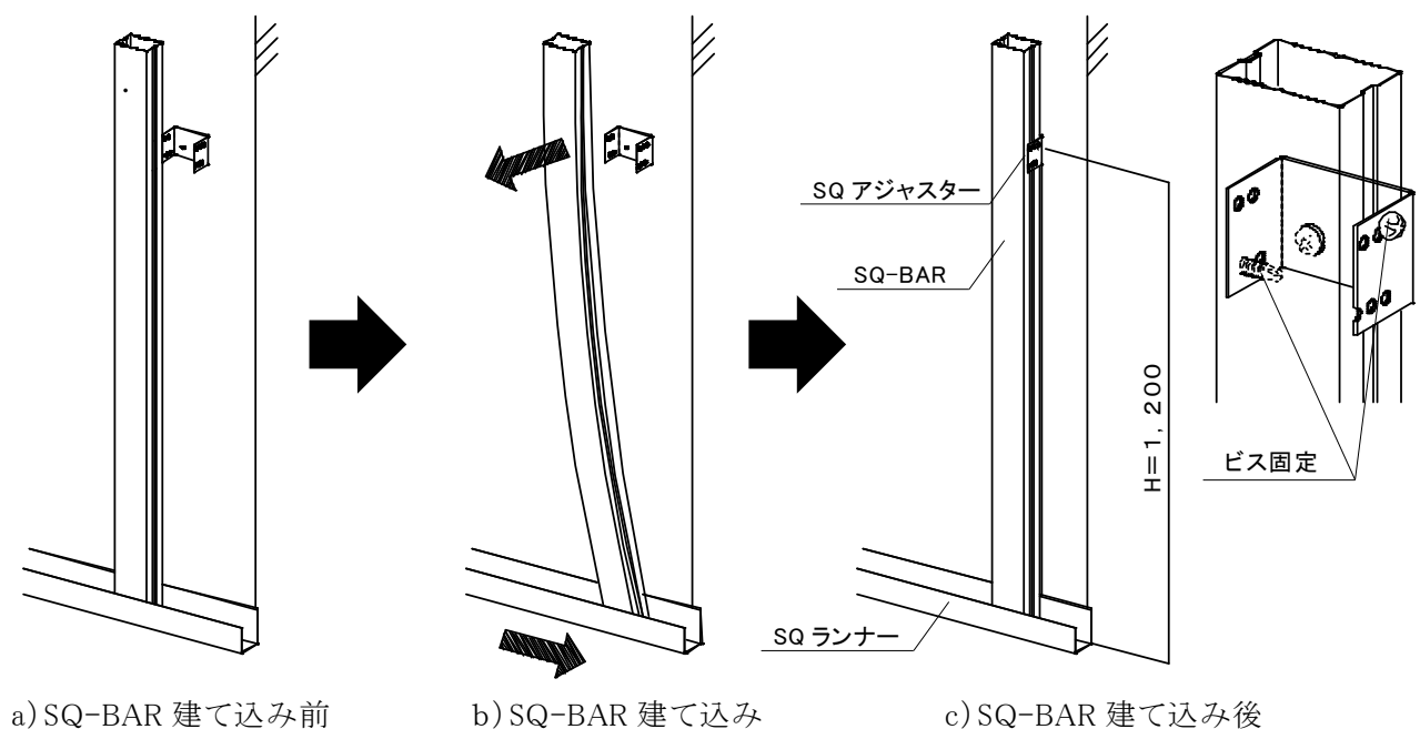
図 2-5-3 SQ アジャスター取付図
