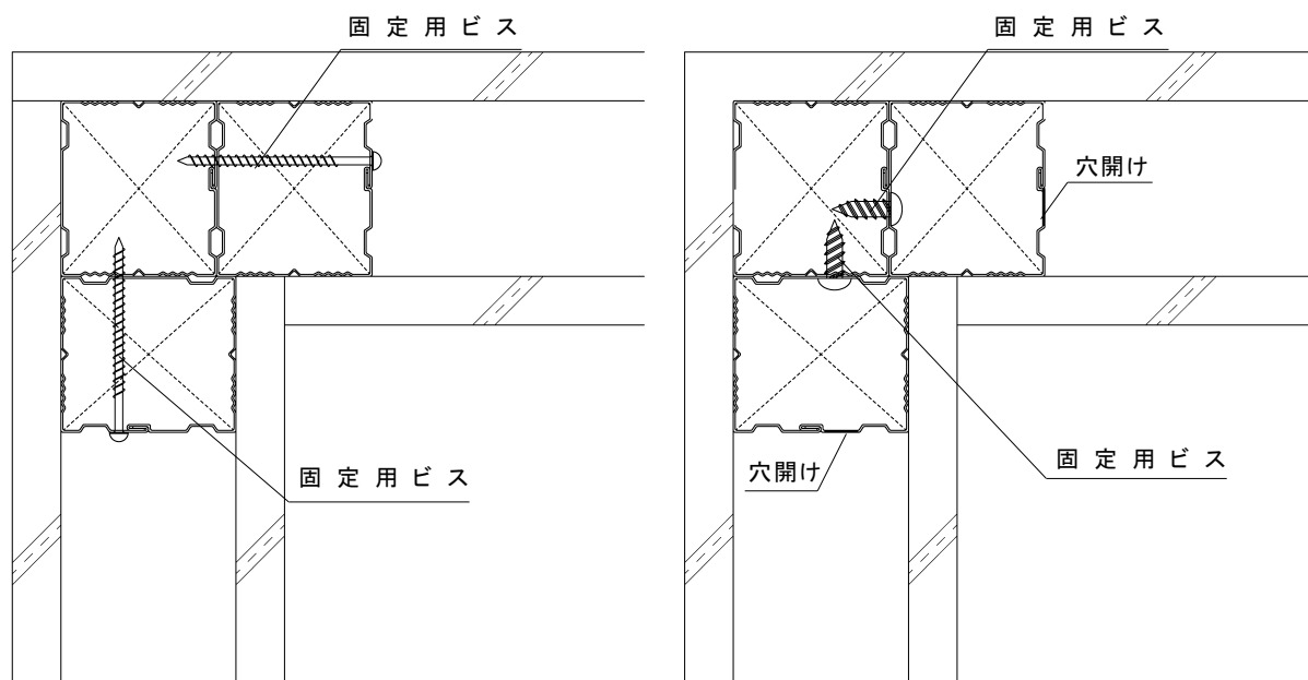
図 3-1-1 (参考)L字コーナー 1
