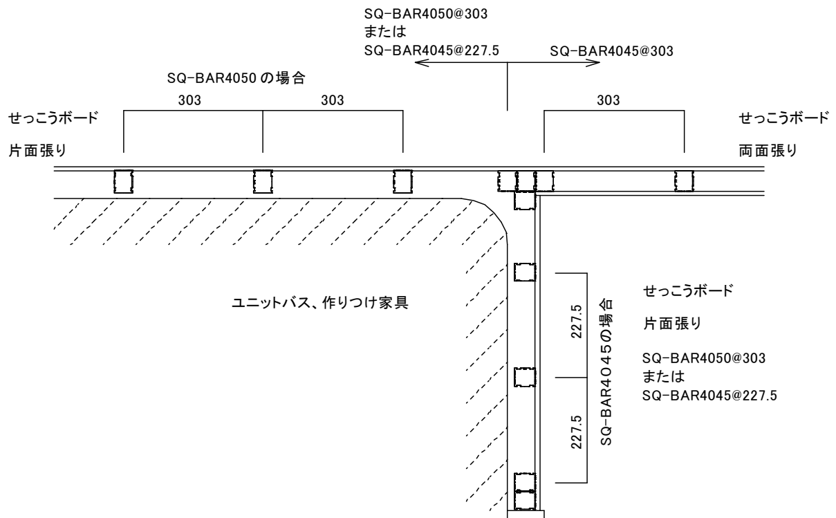
図 3-5-1 (参考)ユニットバス廻り等の片面壁
