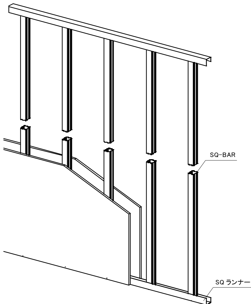
図 1-2-1 SQ 壁工法(例図)
