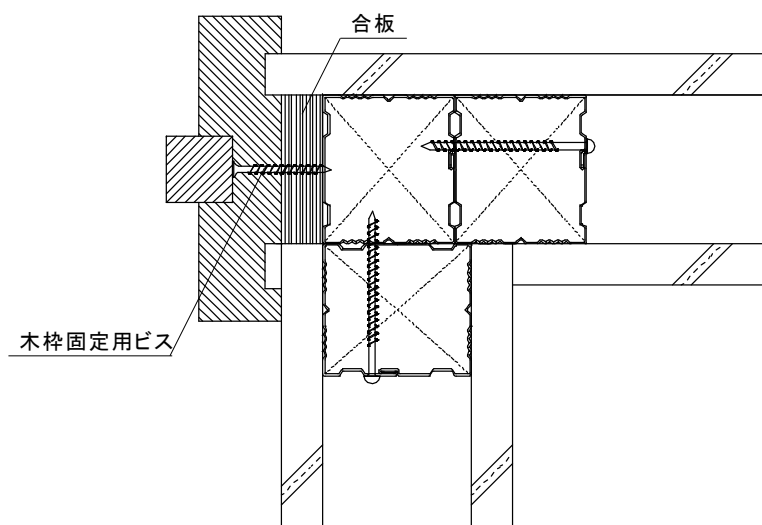
図 3-1-2 (参考)L字コーナー 2
