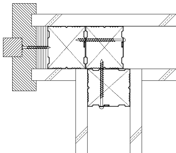
図 3-2-2 (参考)T 字コーナー 2
