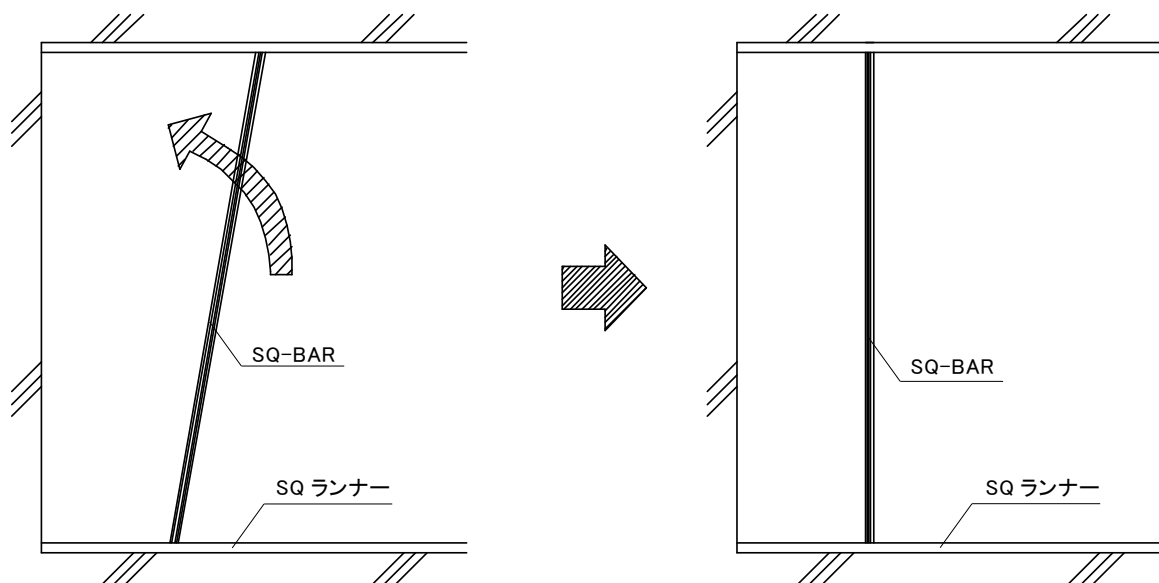
図 2-3-1 SQ-BAR の建て込み
