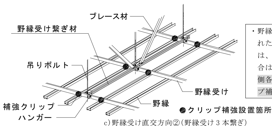
図 2-5-11 クリップ補強の施工箇所
