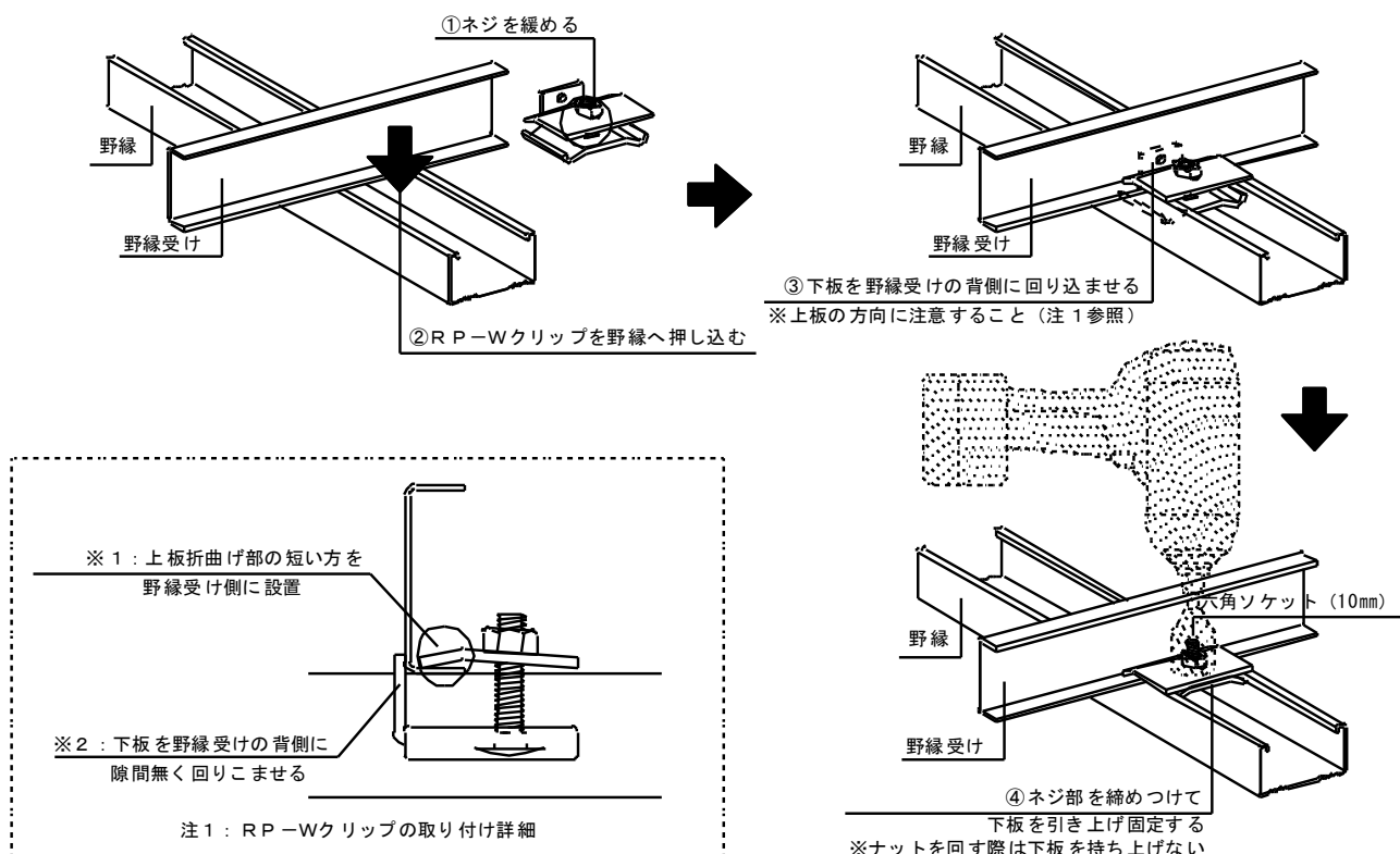
図 2-4-1 RP-Wクリップの施工方法
