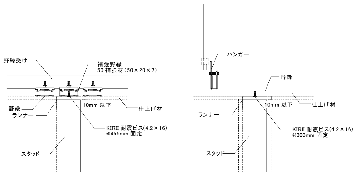
図 3-4-1 (参考例) 天井下間仕切りの接合方法 JIS19 形仕様
