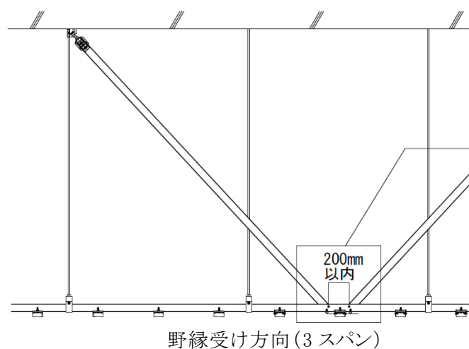
図 2-5-10 ブレース取付け例②
