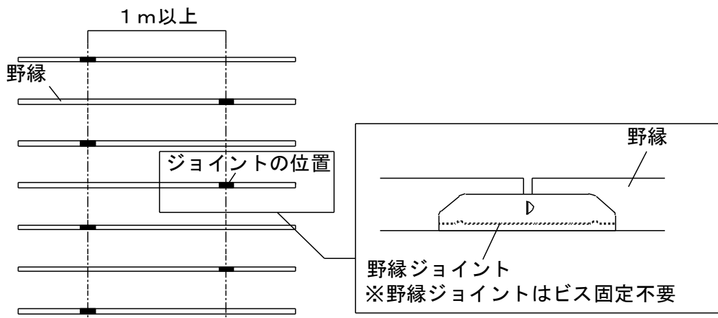
図 2-4-2 野縁の継手
