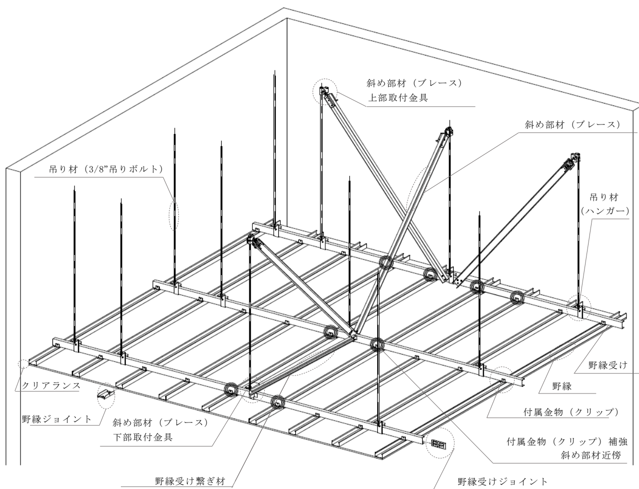
図 1-2-1 新耐震 FullPower 天井 (JIS19 形・JIS25 形仕様) (例図)
