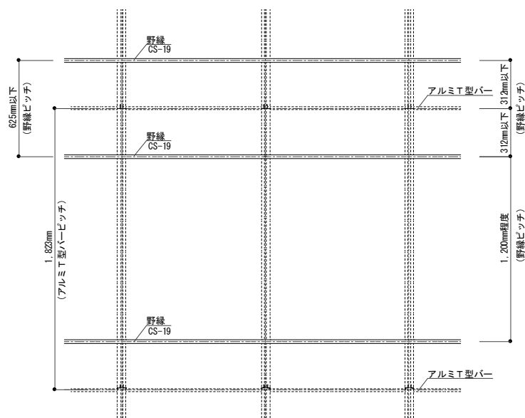
図 2-4-2 野縁の配置
