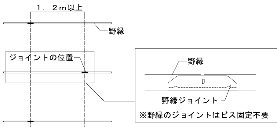
図 2-4-3 野縁の継手
