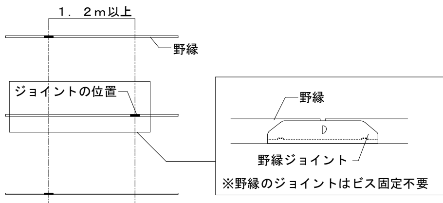
図 2-4-3 野縁の継手
