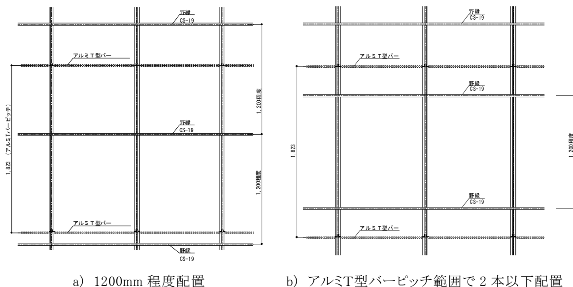
図 2-4-2 野縁の配置
