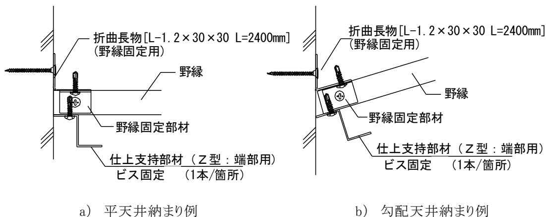
図 2-7-3 仕上支持部材(Z型:端部用)の設置
