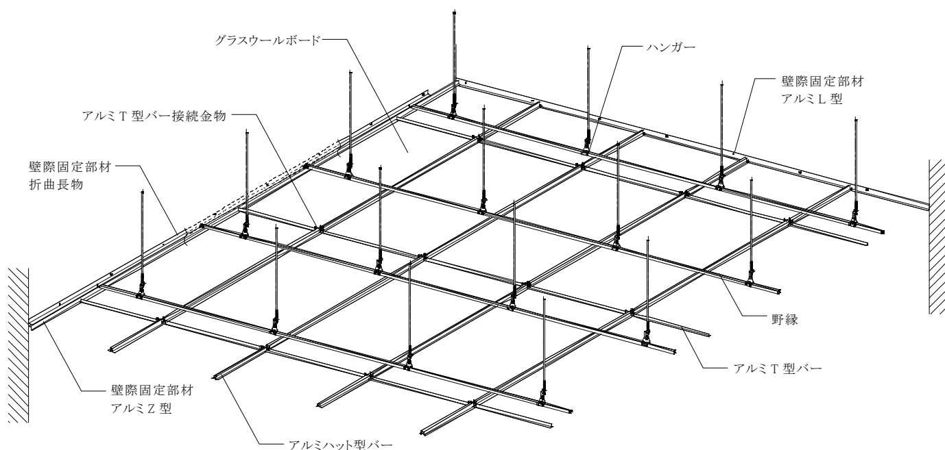
図 1-2-1 安心天井 S (例図)
