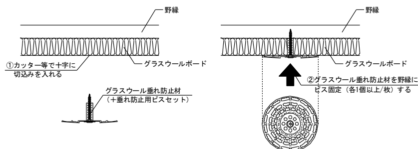
図 2-10-1 グラスウール垂れ防止材の設置
