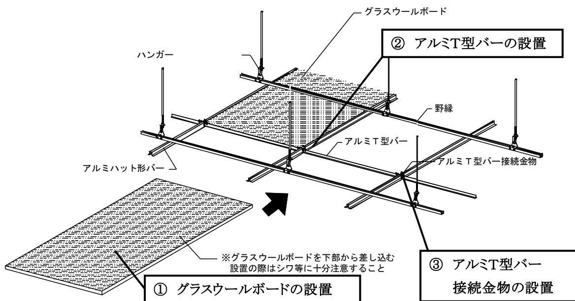
図 2-11-2 グラスウールボードの設置手順
