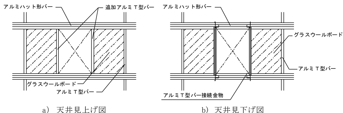
図 3-1-1 開口部の納まり例
