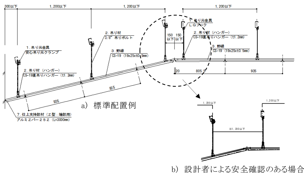
図 2-3-1 吊り材の配置例
