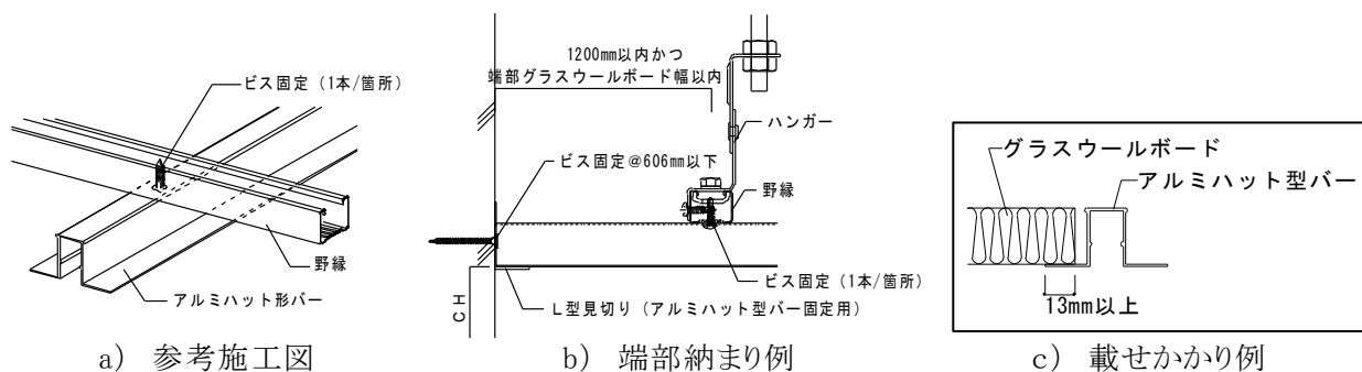
図 2-7-1 野縁とアルミハット型バーの設置
