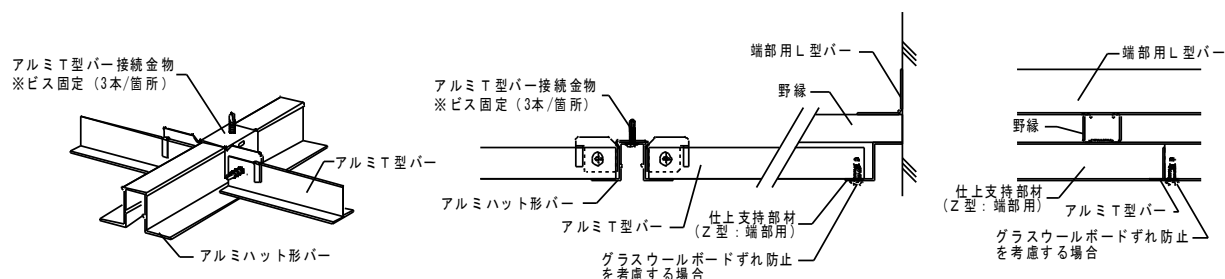
図 2-11-1 アルミT型バーの設置
