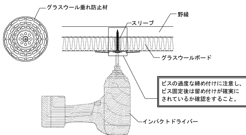
図 2-10-2 グラスウール垂れ防止材の設置注意事項
