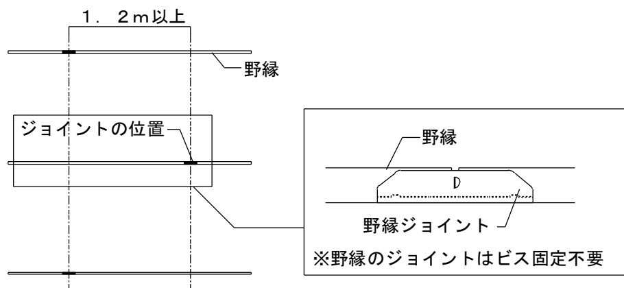
図 2-4-3 野縁の継手
