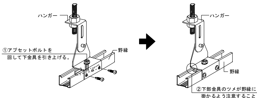
図 2-4-1 ハンガーと野縁の取付け
