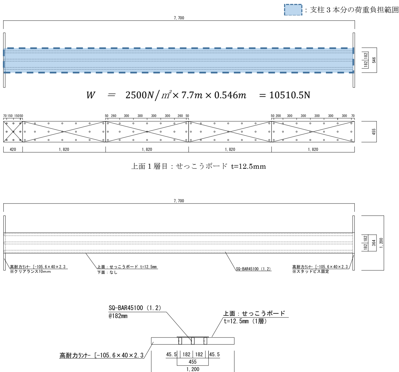
図1 試験体詳細図（平面・断面）
