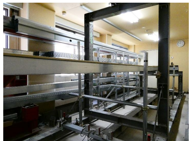
写真 6 試験実施状況 変位計設置
