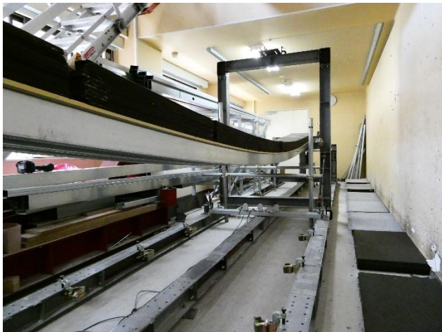
写真 7 最大荷重時 高比重アスファルト系面材設置
