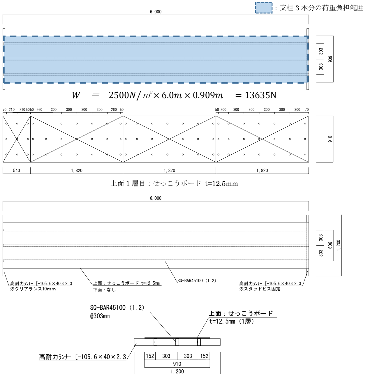
図 1 試験体詳細図 (平面・断面)
