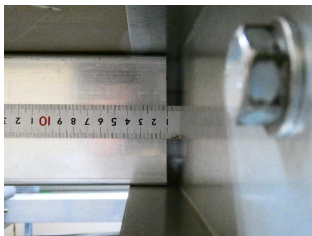
写真 4 試験体施工状況 上部ランナー
