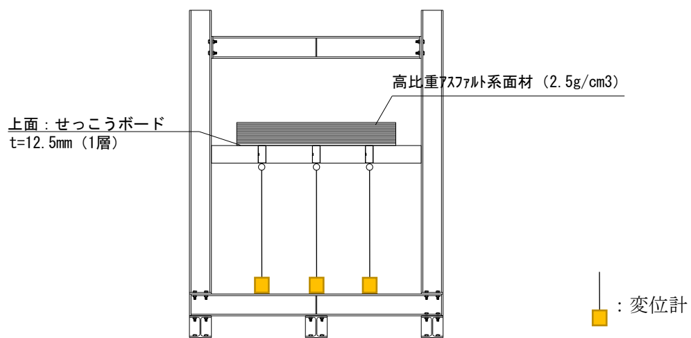
A-A断面図
