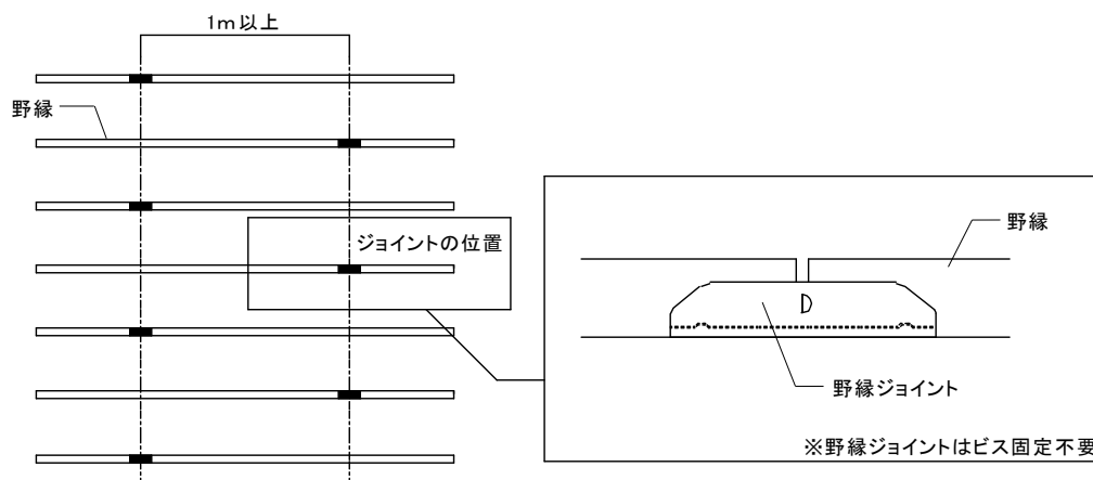
図 3-5-3 野縁の継手
