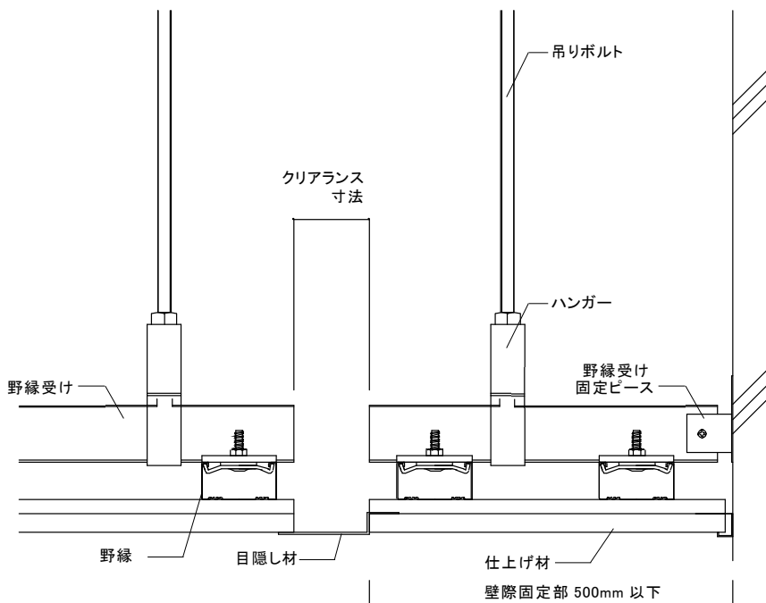
b) スリットを設けた場合
