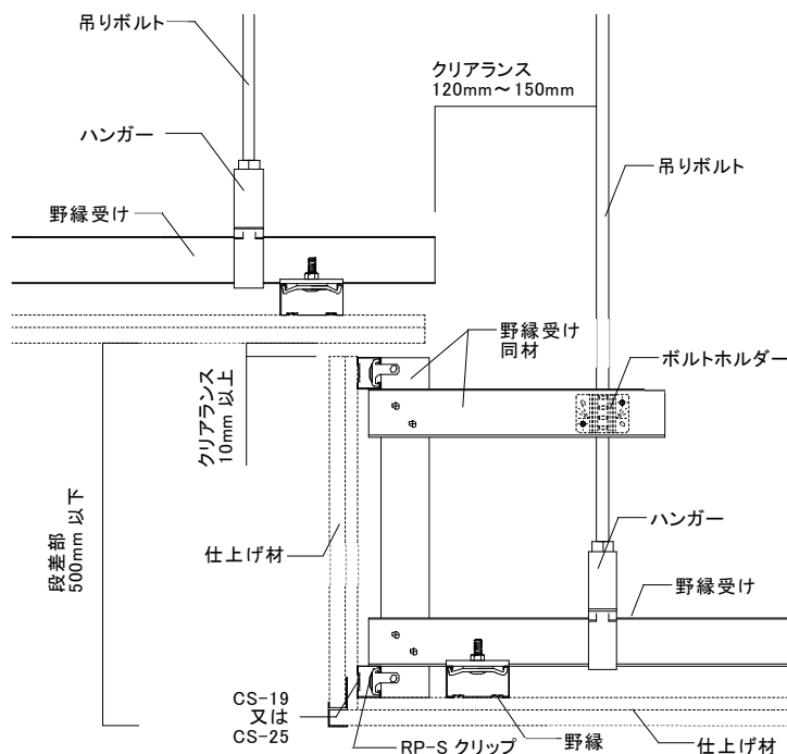
図 2-7-2 (参考例)クリアランスの確認(段差部)
