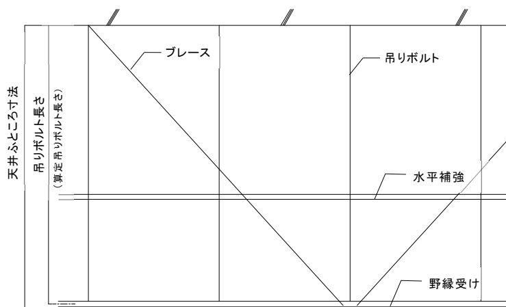
図 5-1-3 ブレース1段の場合(3スパン)
