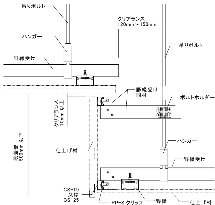
a) 廻り縁を使用した場合
