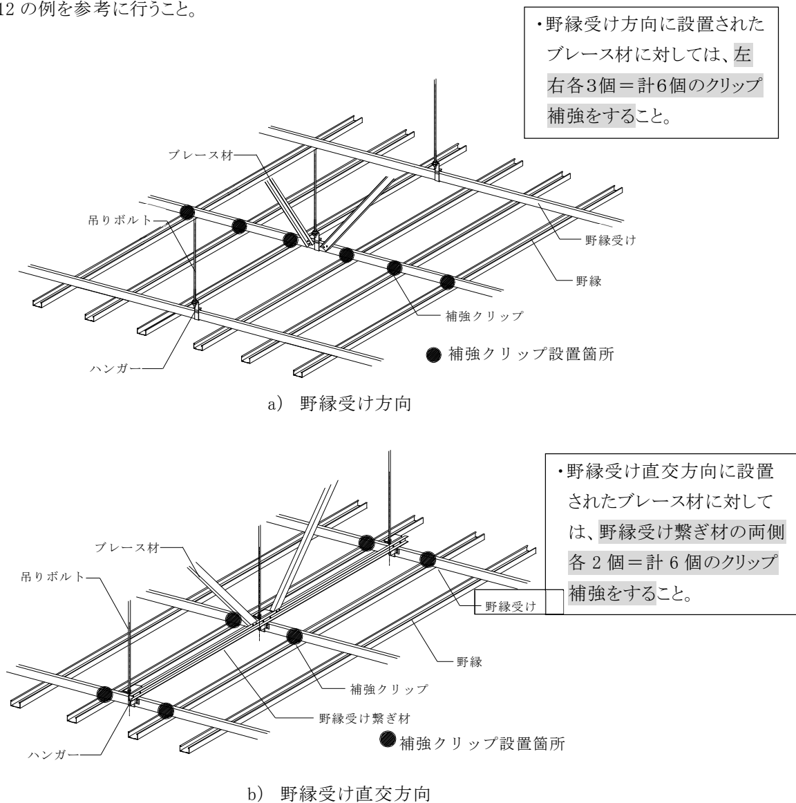
図 2-5-12 補強クリップ設置箇所
