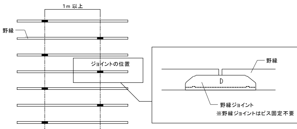
図 2-4-2 野縁の継手
