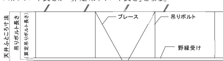
図 5-1-1 ブレース1段の場合(1スパン)
