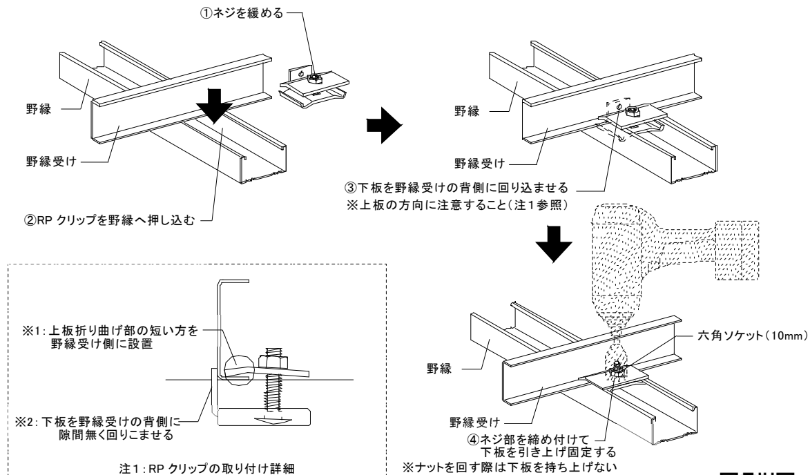
図 2-4-1 補強クリップの施工方法
