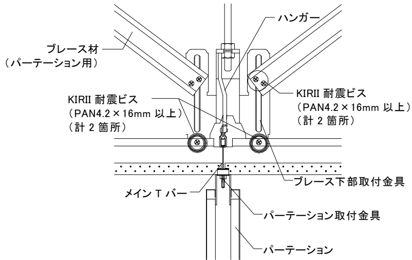
図2-10-1 パーテーション設置部参考納まり
