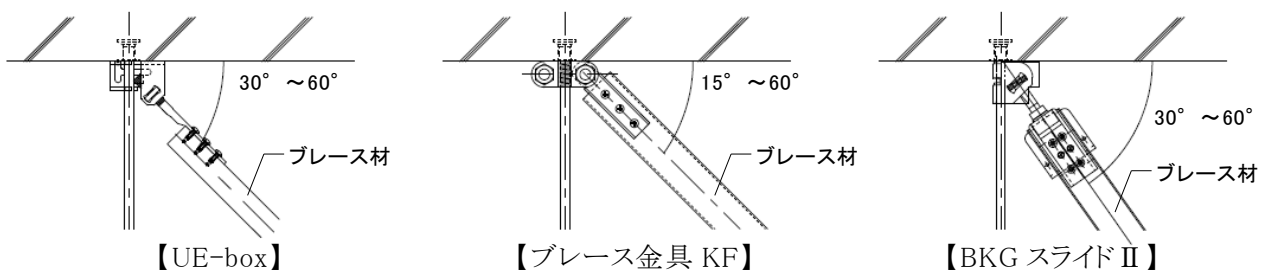
図 2-7-8 ブレース設置角度
