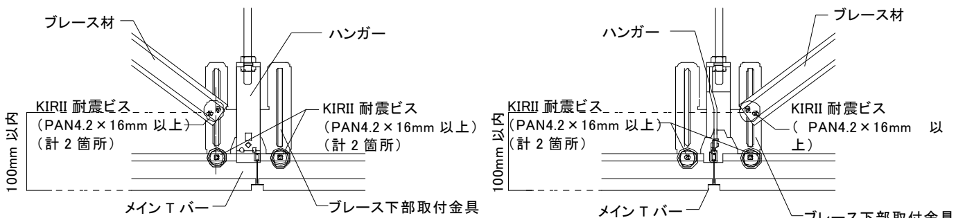
【メイン T バー方向】
