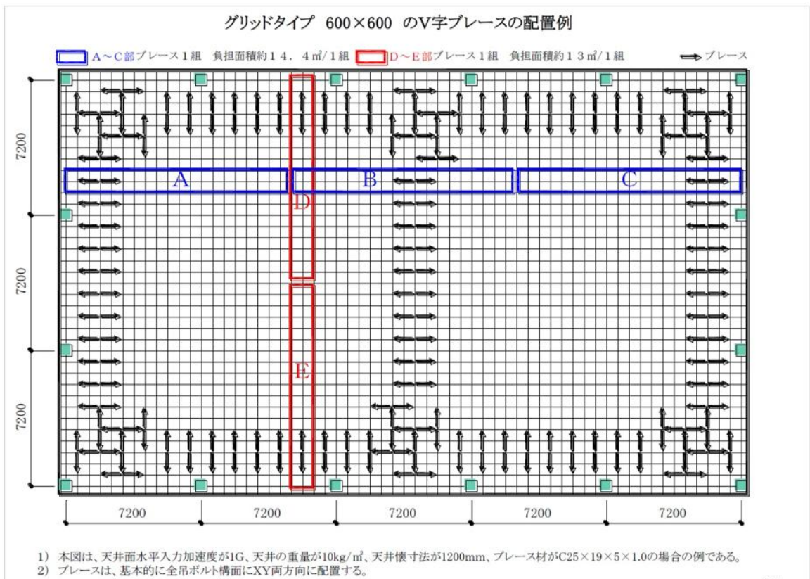
d) プレースの配置例(V字)
