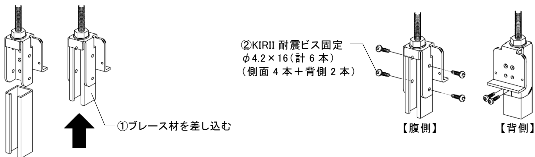
a) 【種別①】万能キャッチャーボルト 70 の施工方法
