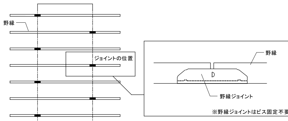
図 2-4-2 野縁の継手
