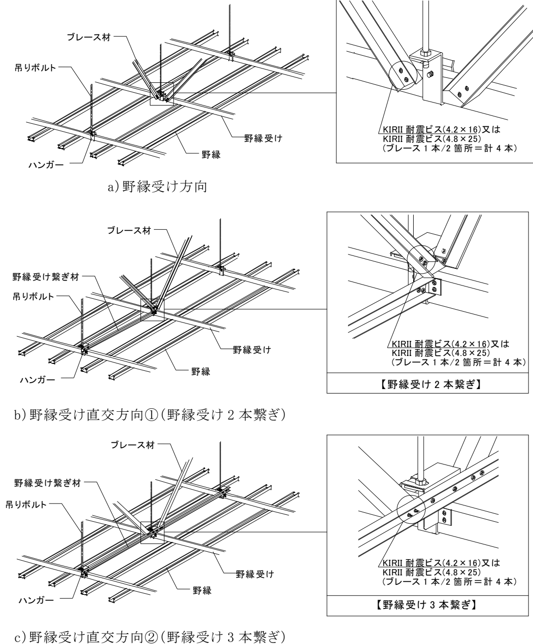
図 2-6-7 ブレース下部取付詳細
