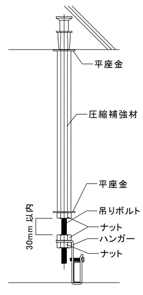
図 2-2-4 圧縮補強材全体納まり
