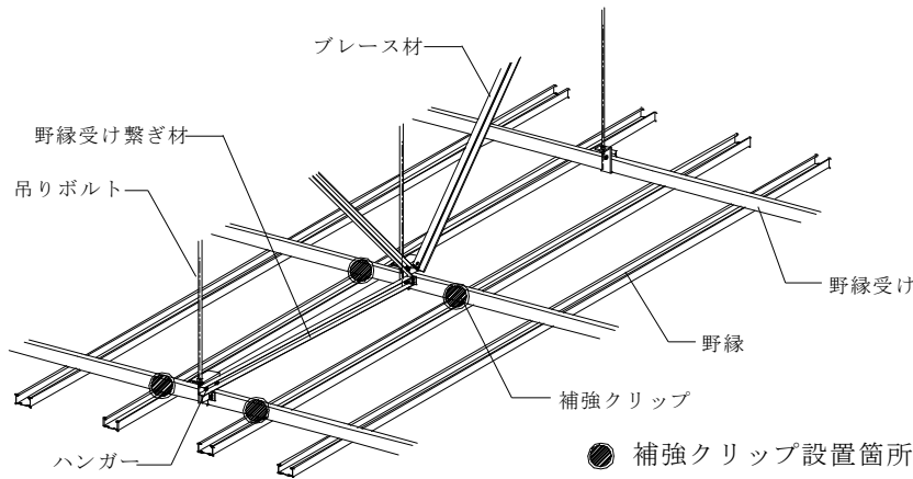
b) 野縁受け直交方向①(野縁受け 2 本繋ぎ)
