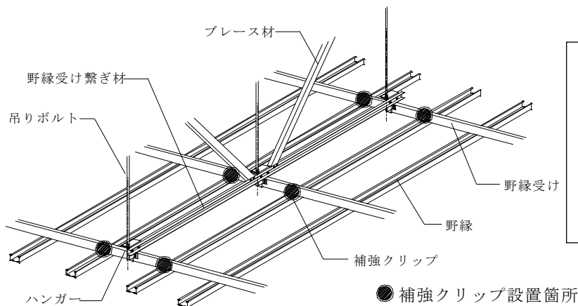
c) 野縁受け直交方向②(野縁受け 3 本繋ぎ)
