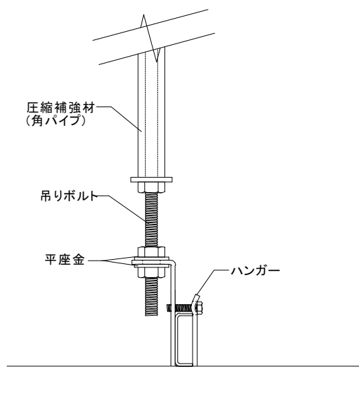
図 2-2-6 ハンガー取付詳細
