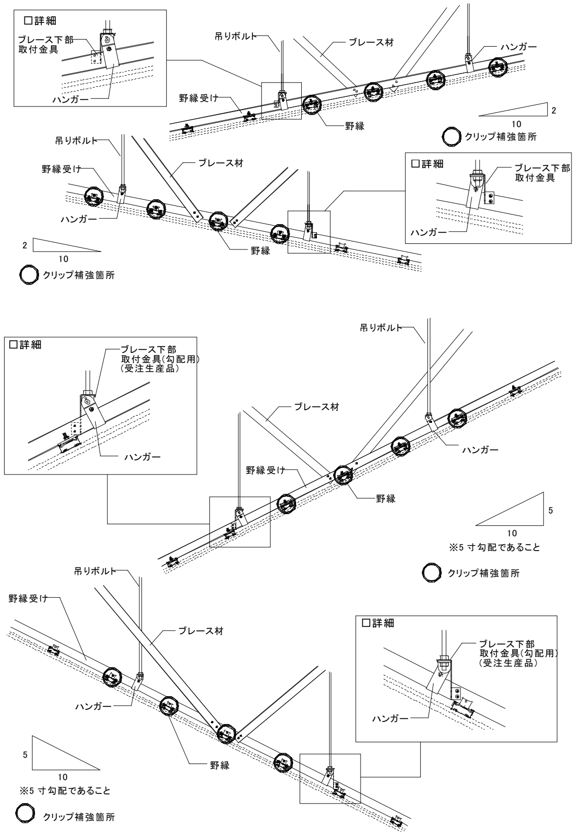
図 2-8-1 (参考例) 勾配天井施工例(野縁受け方向)
