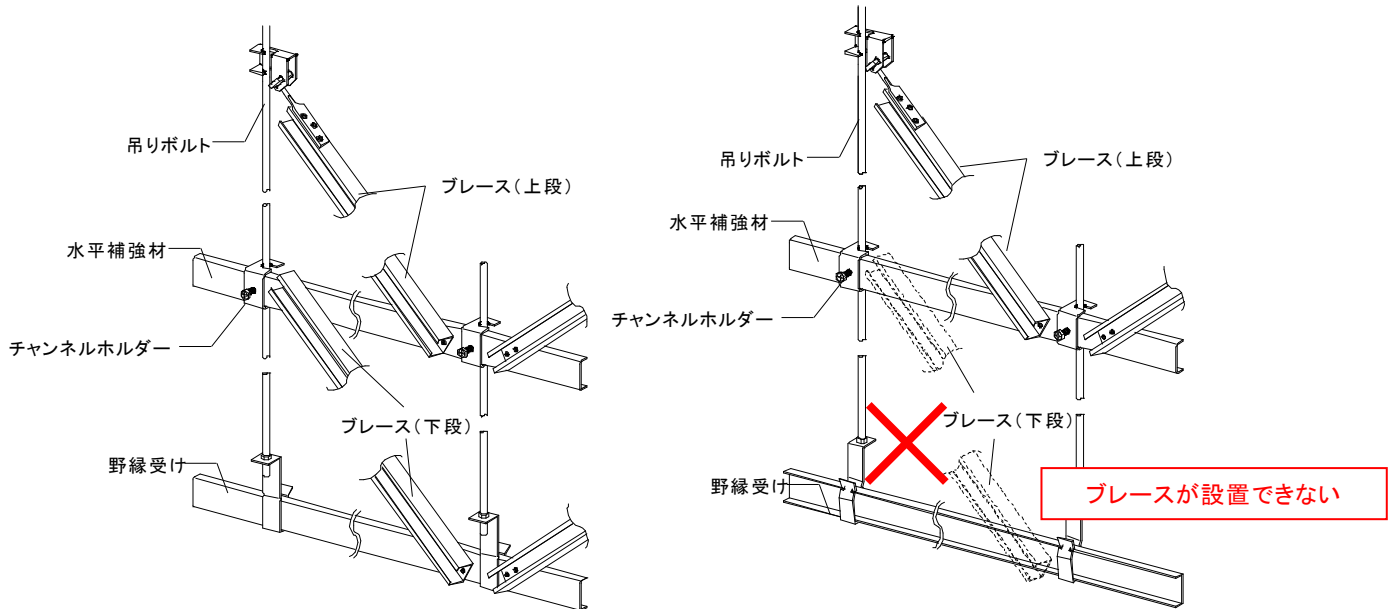
a)水平補強と野縁受けの向きが同じ場合
