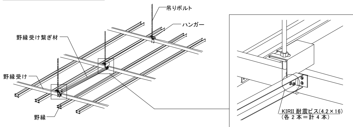
a) 野縁受け 2 本繋ぎ
