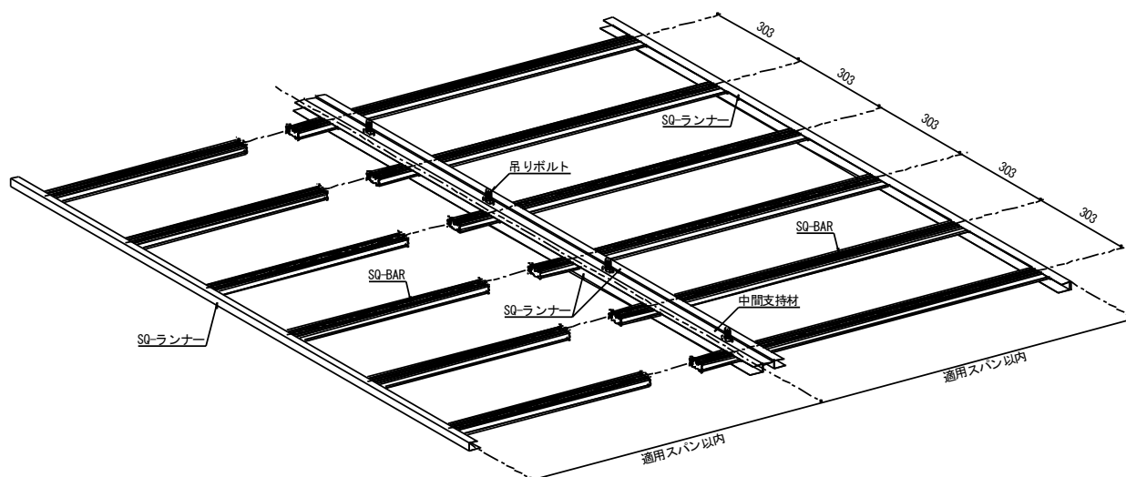
図 1-2-1 SQスリムシーリング (例図)
