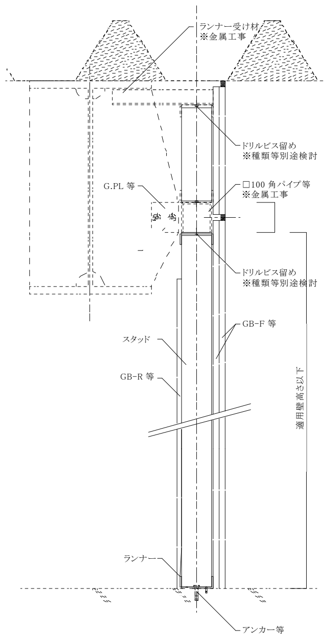
図 3-4-1 (参考例)適用壁高さを超える場合
