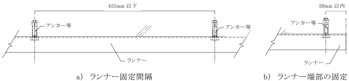
図 2-2-1 ランナーの固定間隔
