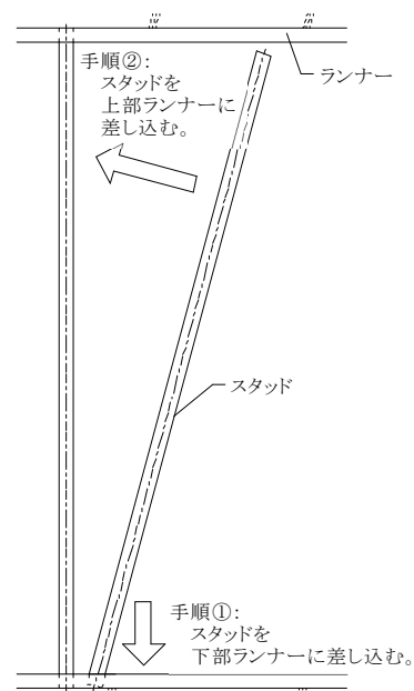
b) スタッドの立上げ
