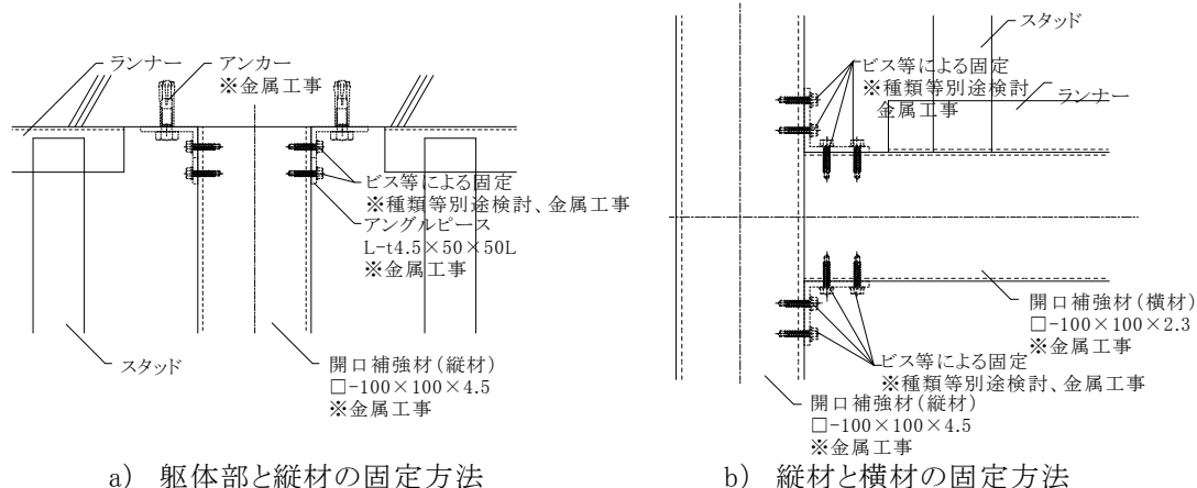
図 3-3-2 (参考例)開口部の補強詳細
