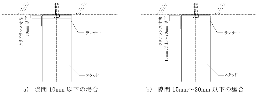
図 2-3-1 上部ランナーとスタッドの隙間
