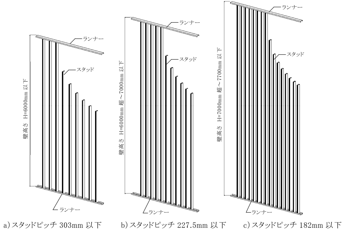
図1-2-1 SQ-WALL2500 工法(ソリーダ)(例図)
