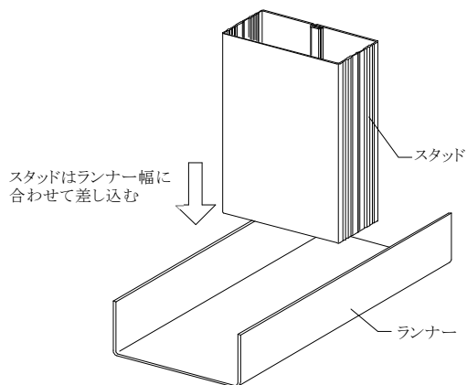
a) 下部ランナーへの差し込み
