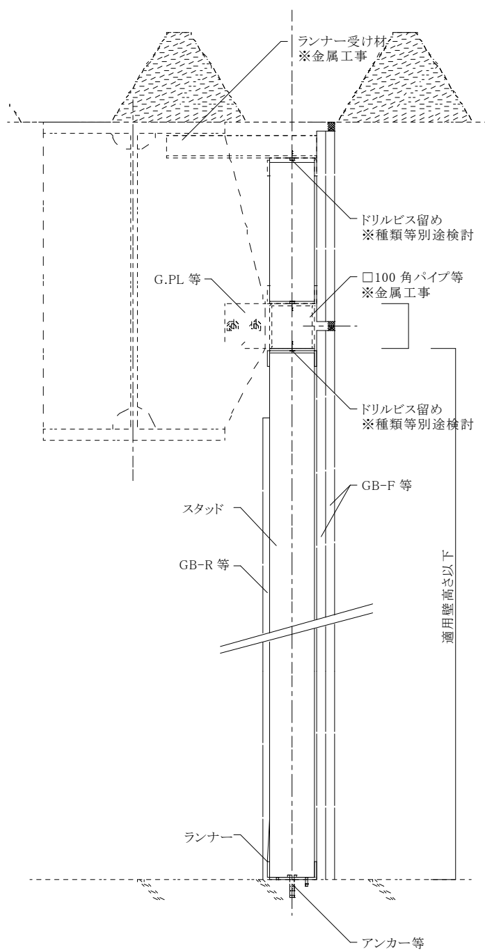
図 3-4-1 (参考例) 適用壁高さを超える場合
