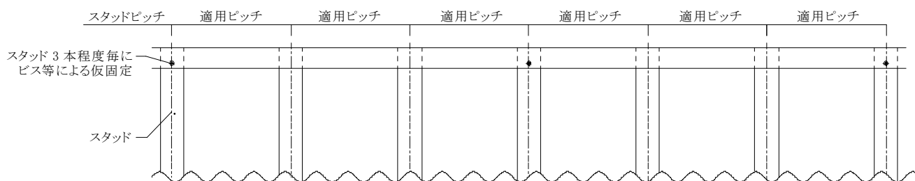
図 2-4-2 スタッド滑動防止の仮固定
