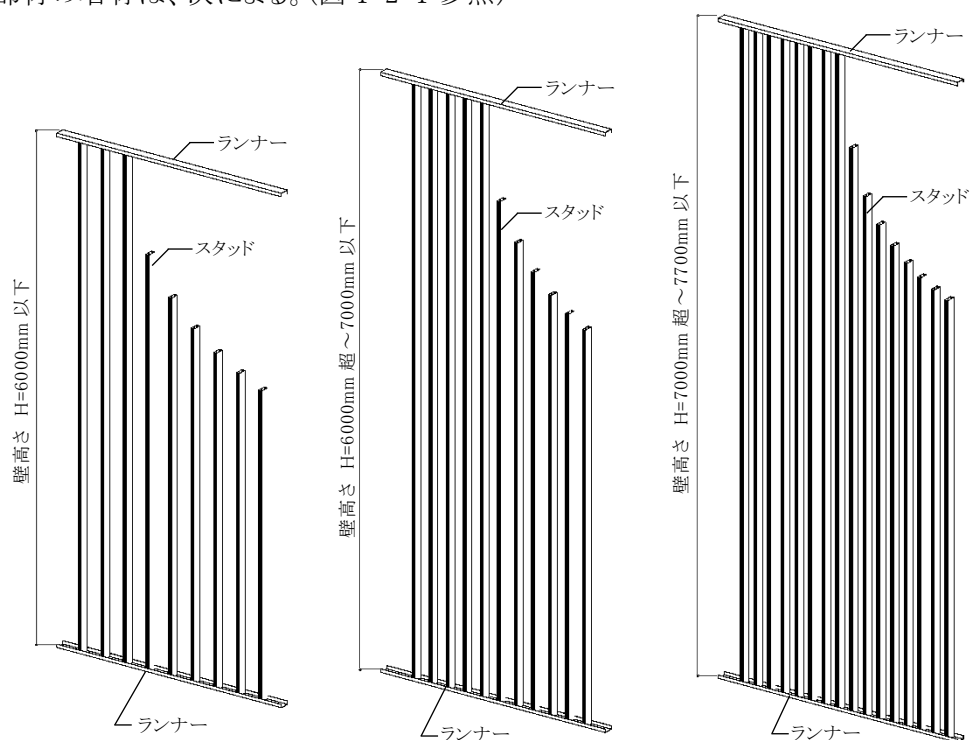
a) スタッドピッチ 303mm 以下 b) スタッドピッチ 227.5mm 以下 c) スタッドピッチ 182mm 以下
