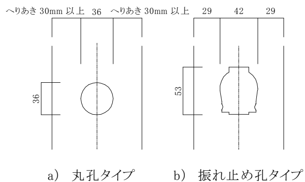
図 2-5-2 貫通孔の種類
