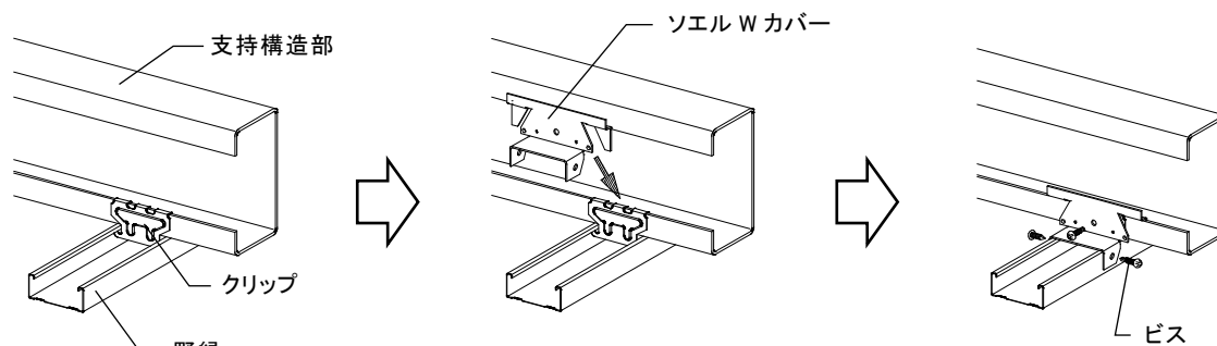
図 2-2-1 ソエル W カバーの施工方法
