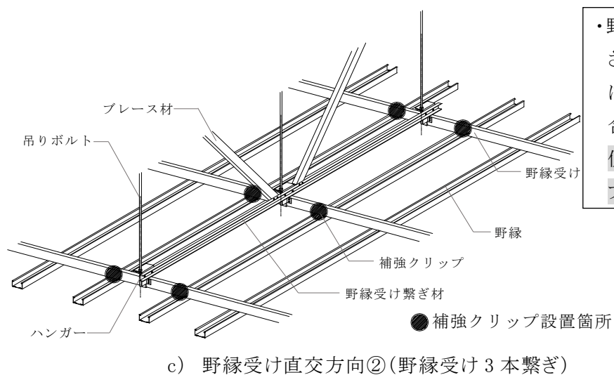
図 2-6-12 補強クリップ設置箇所
