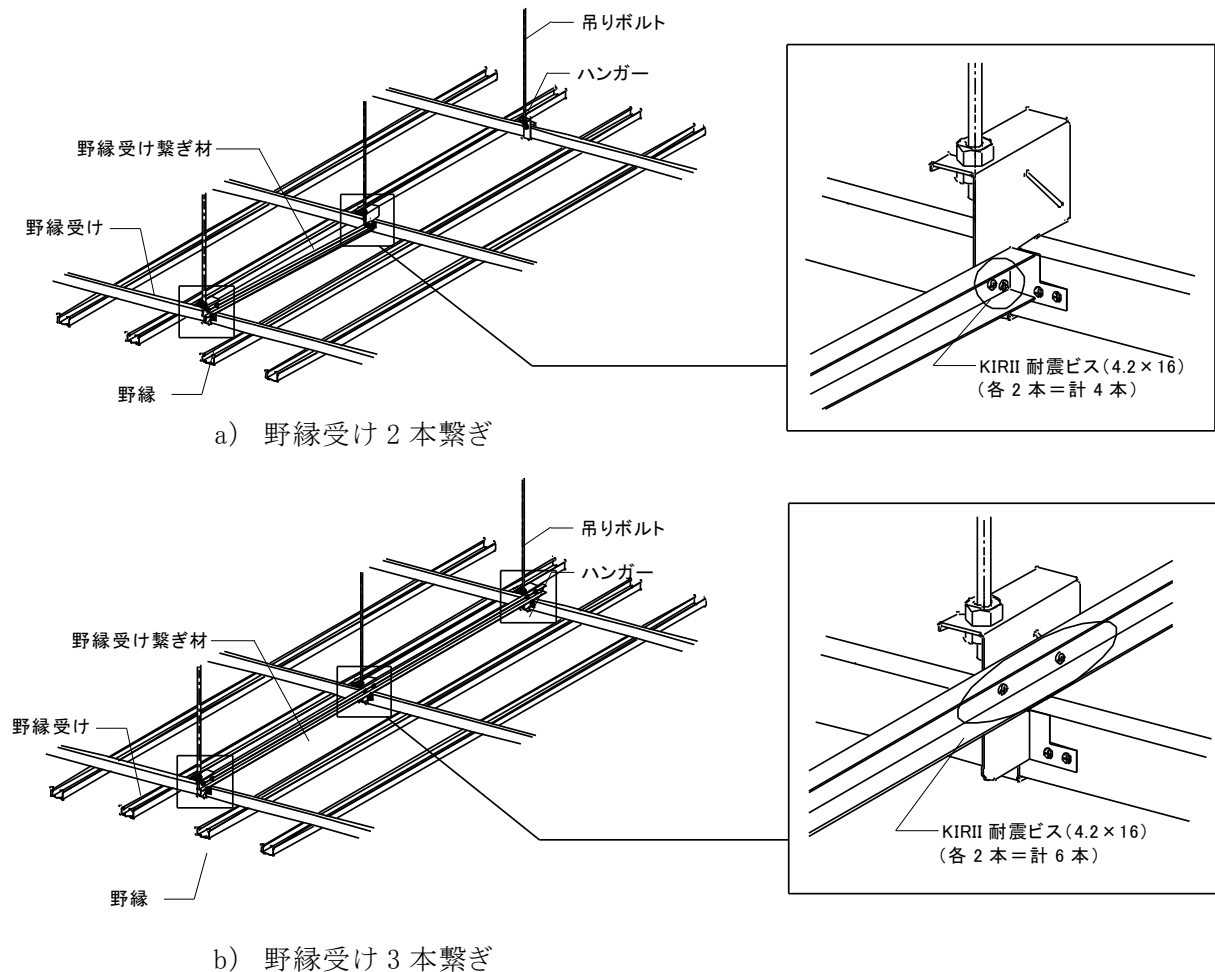
図 2-6-2 野縁受け繋ぎ材の設置
