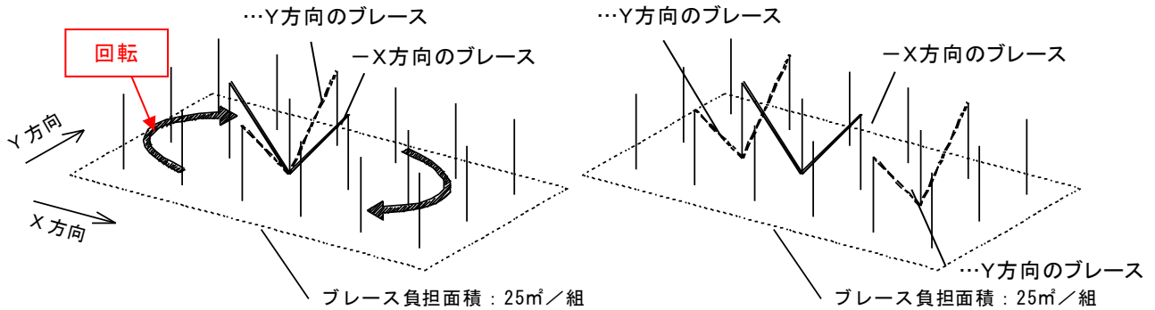
a) 天井中央のみにブレースを設置
