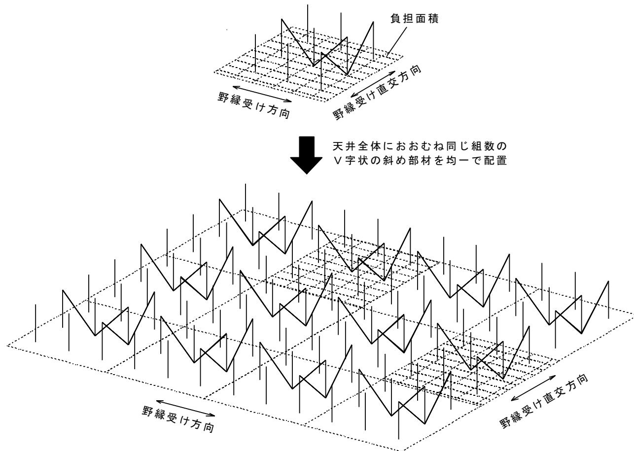
図4-1-1 (参考例)負担面積内のブレース
