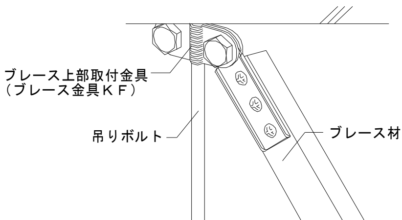
図 2-5-5 ブレース上部取付け詳細②
