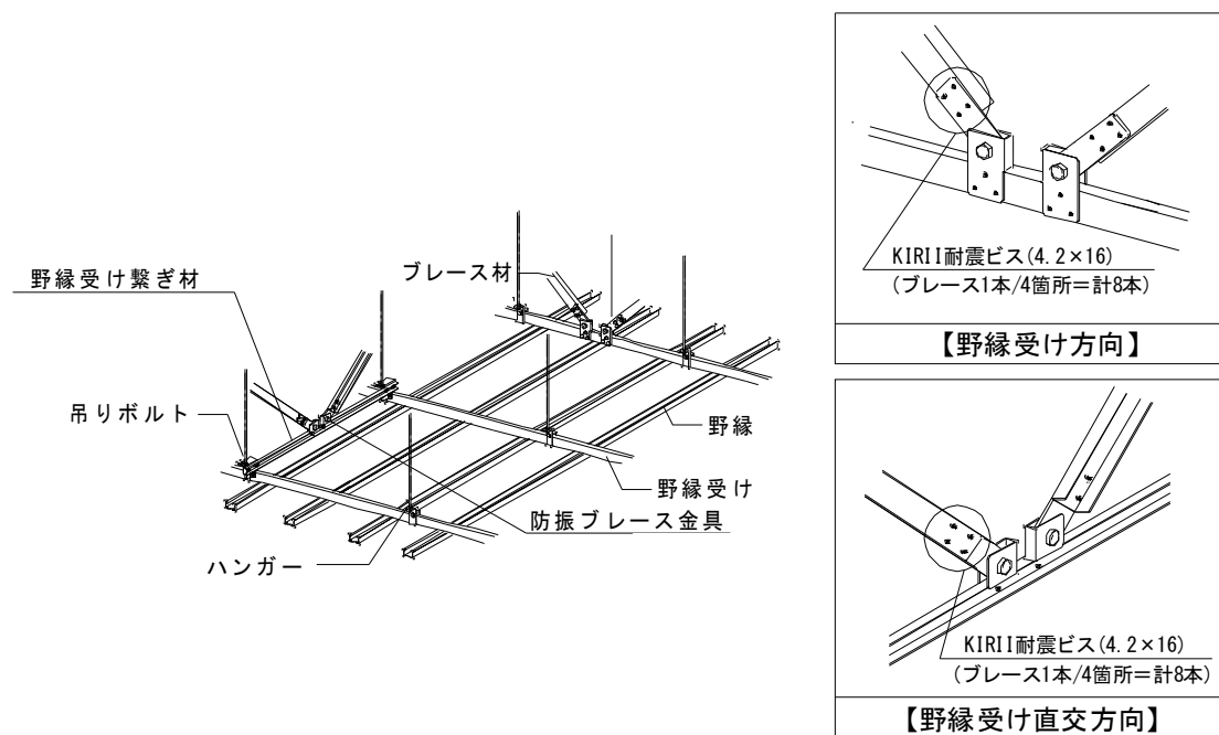
b) ブレース頂点が吊りボルトピッチの中間にくる場合 (ブレース取付 1 スパン・3 スパン)
