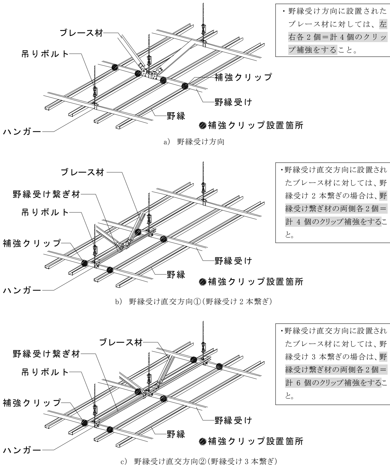
図 2-5-11 補強クリップ設置箇所
