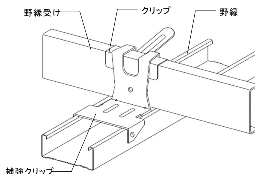
図2-4-2 壁面と接する周辺部のクリップ
