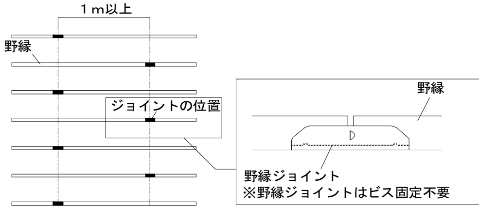
図 2-4-3 野縁の継手
