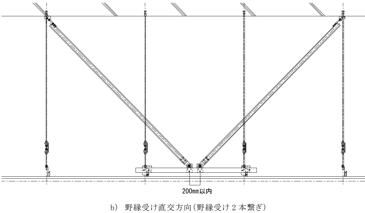
図 2-5-10 ブレース取付け例②
