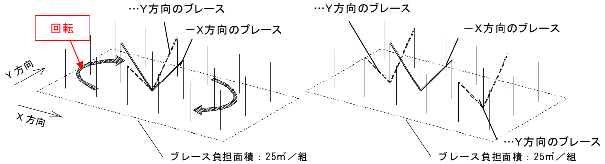
図 4-2-1 中小規模の空間の天井に設置されるブレース
