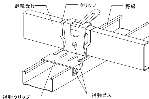
図2-4-1 補強部のクリップ
