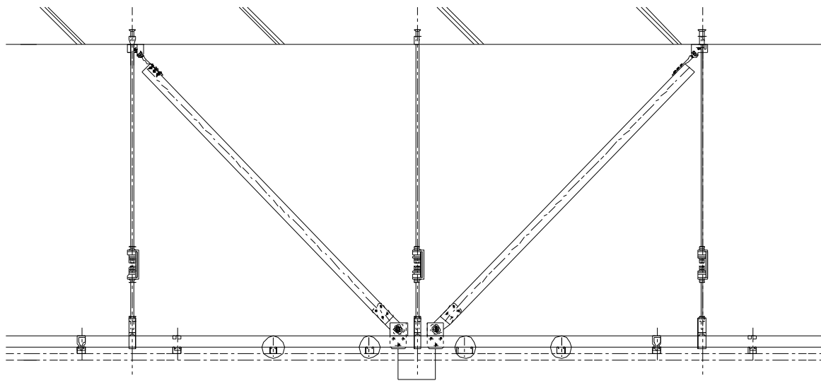
a) 野縁受け方向
