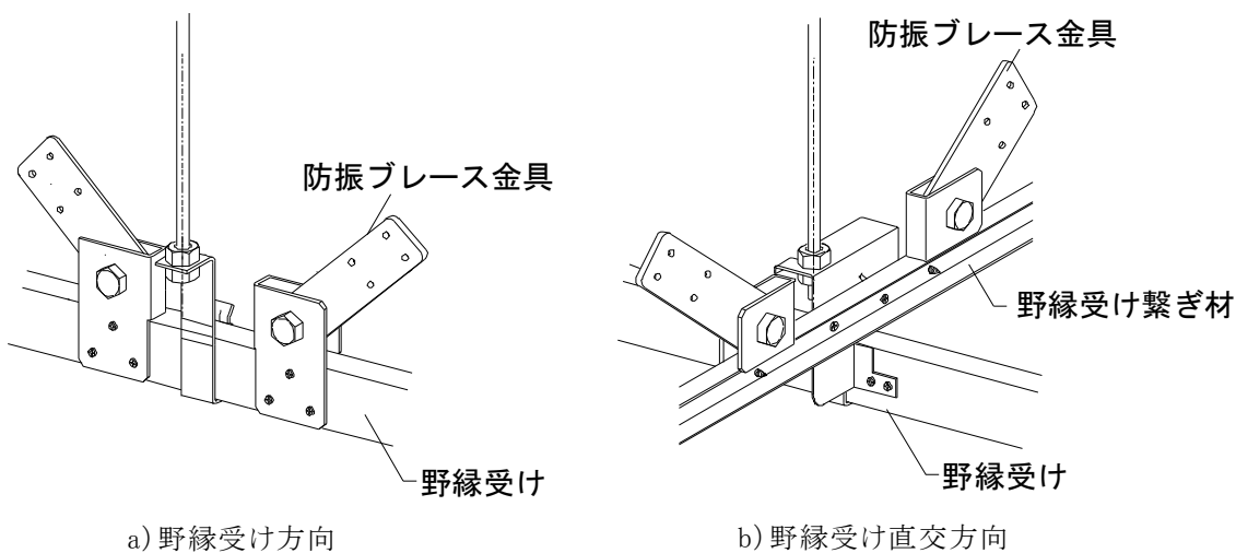
図 2-5-3 防振ブレース金具の取付け
