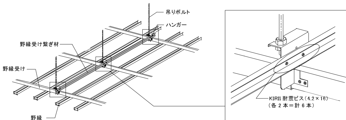
図 2-5-2 野縁受け繋ぎ材の設置
