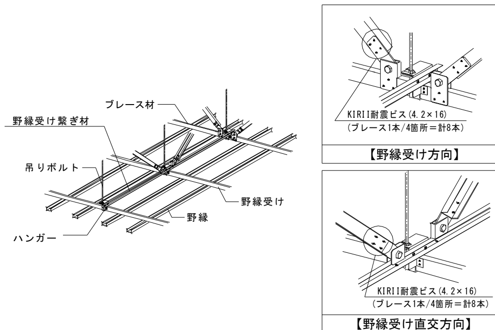
a) ブレース頂点が吊りボルトの両側にくる場合 (ブレース取付 2 スパン・4 スパン)
