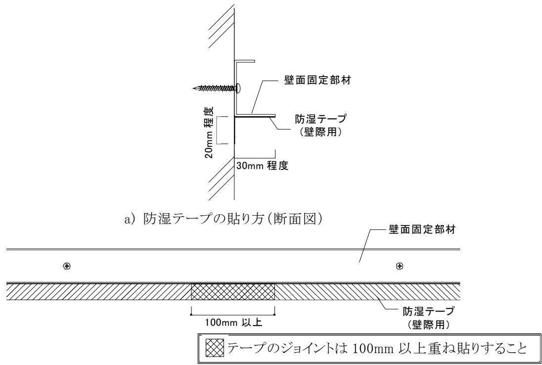
図 2-3-2 防湿テープの設置状況
