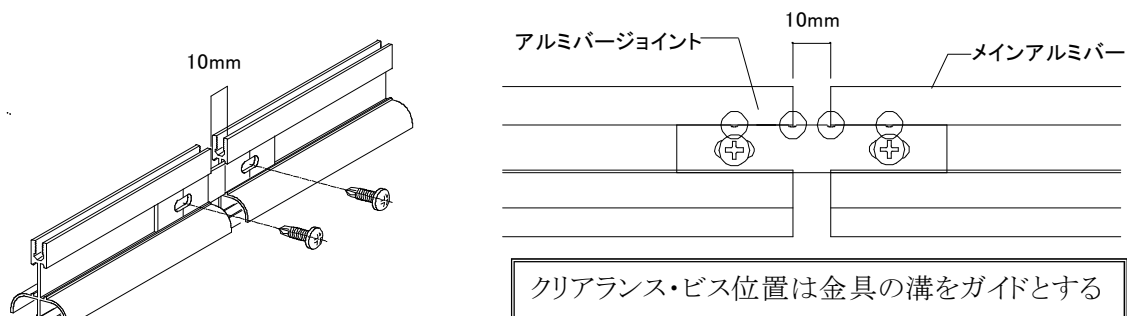
図 2-7-5 アルミバージョイントの施工
