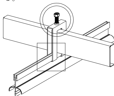
図 2-7-1 クリップの施工状況
