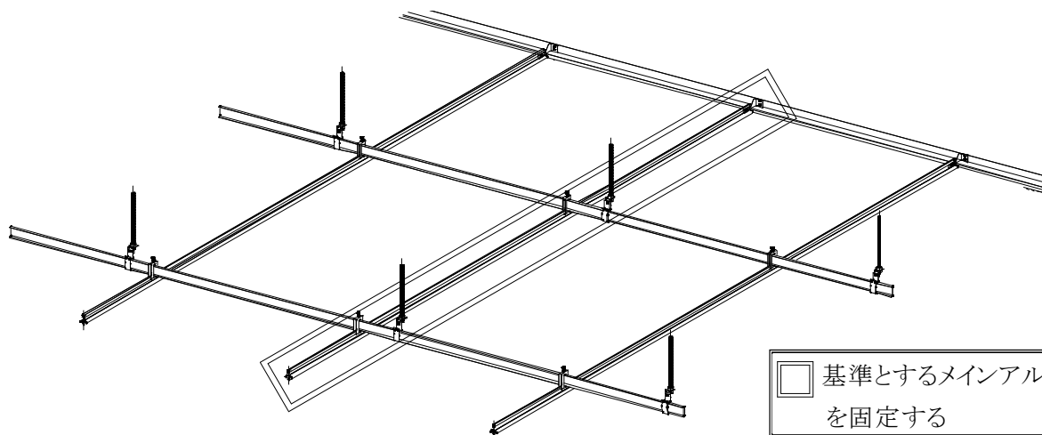
図 2-7-2 基準とするメインアルミバーの固定
