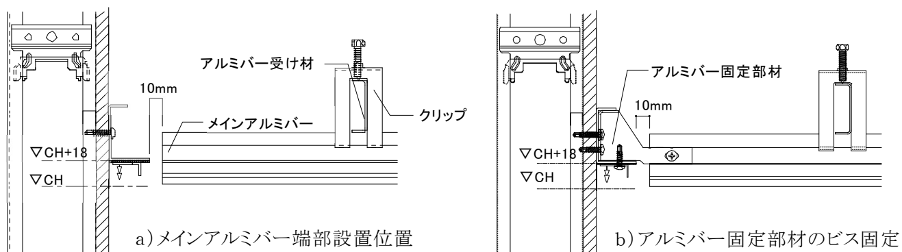
図 2-7-4 アルミバー端部固定部材の設置状況 (壁面が軽量鉄骨の場合)
