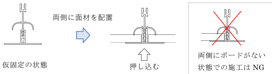
図 2-8-1 軽量不燃ボードの固定手順
