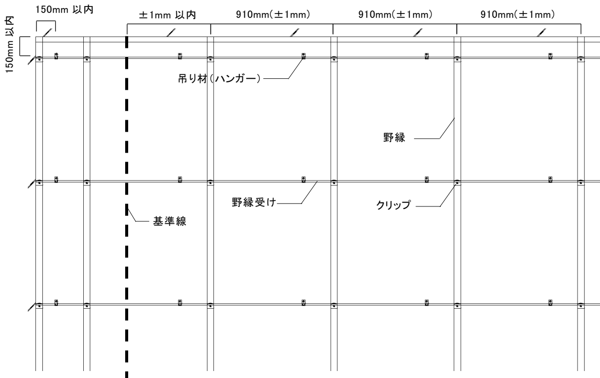
図2-5-1 野縁の配置
