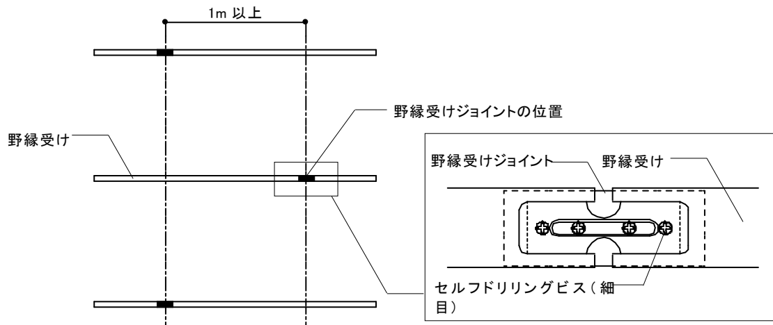
図2-4-2 野縁受けの継手
