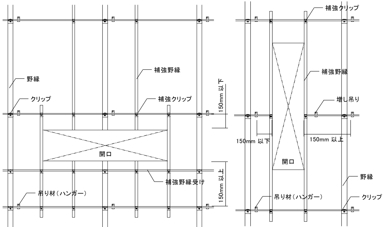
b) 開口部補強例(野縁が切断される場合)
