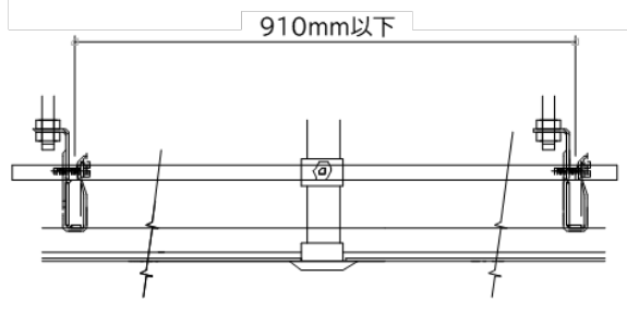
●野縁受け方向断面図
