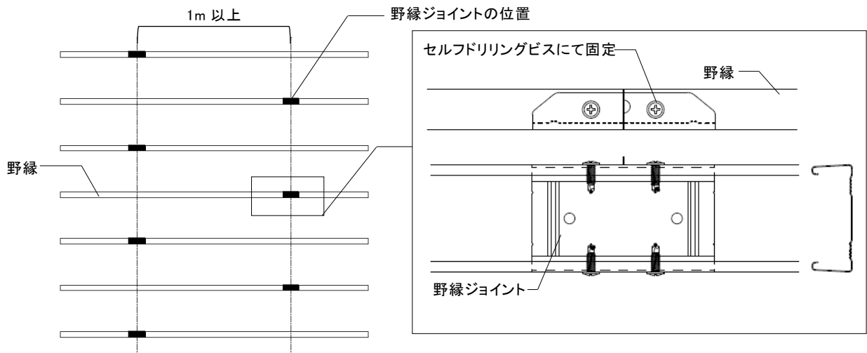
図2-5-3 野縁の継手
