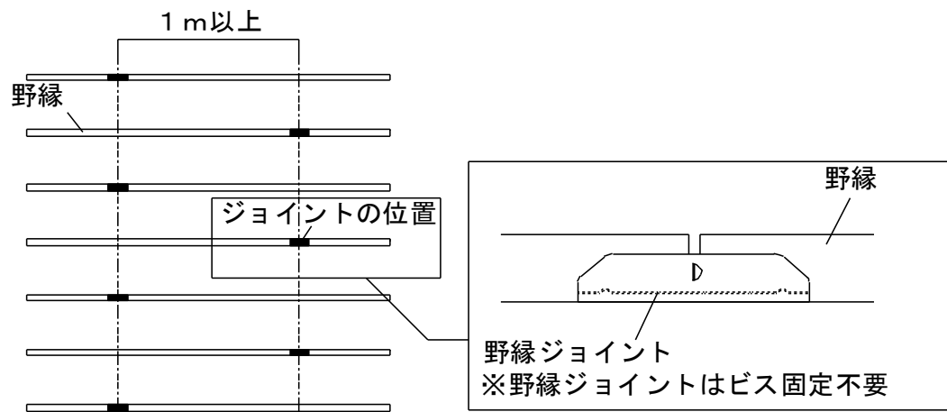
図 3-6-3 野縁の継手
