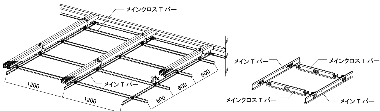
図2-6-2 メインクロスTバーの設置
