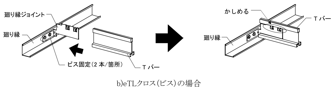
図2-7-1 Tバーと廻り縁の接続
