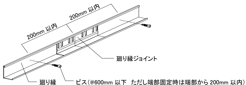
図2-3-2 廻り縁端部のビス固定位置
