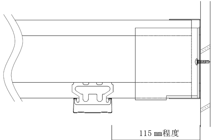
図 2-5-2 端部野縁の取付け箇所
