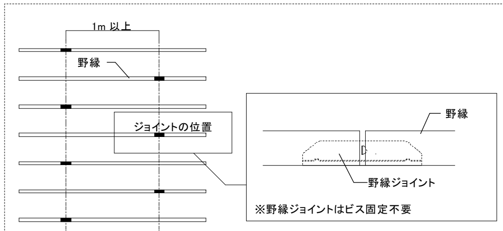
図 2-5-3 野縁の継手
