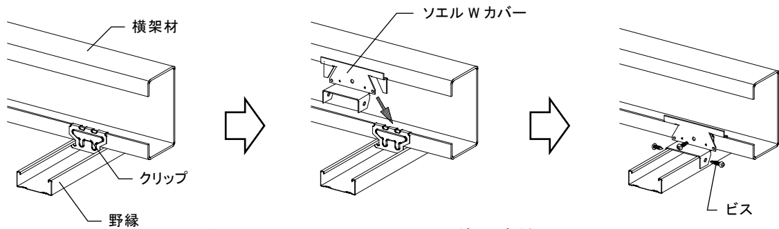
図 2-6-1 ソエル W カバーの施工方法
