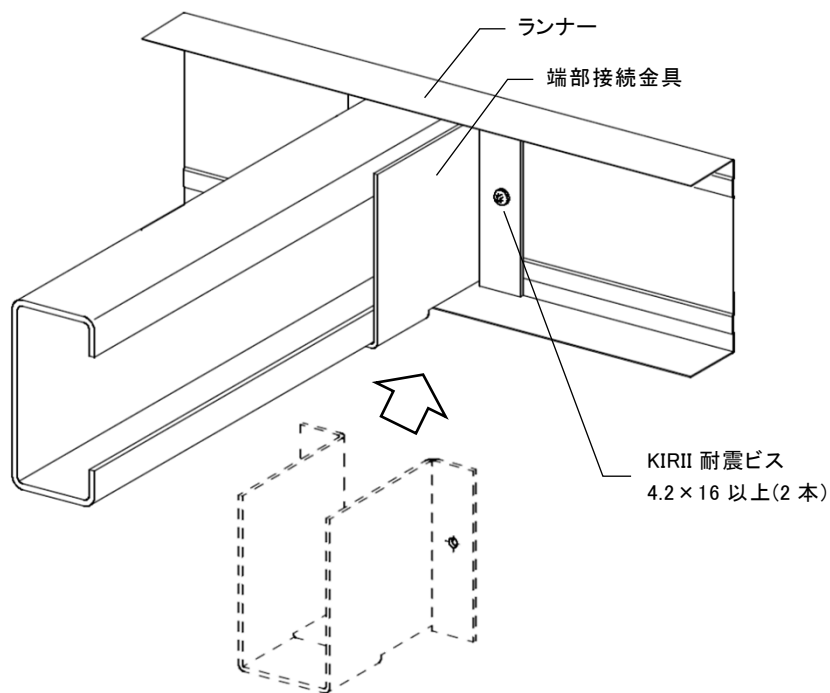
図 2-4-2 端部接続金具の取付け
