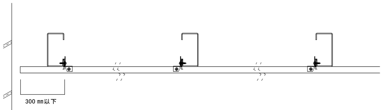
図 2-3-2 横架材端部の向き
