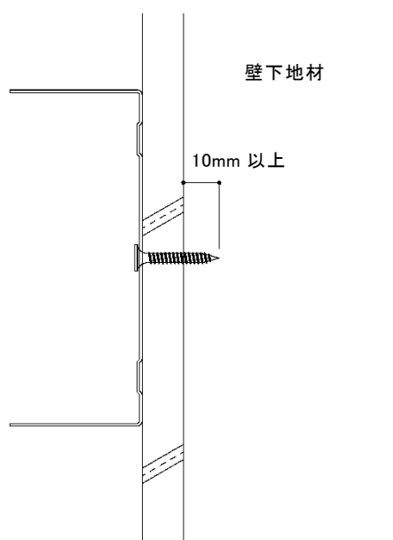
図 2-2-1 ランナー固定部詳細
