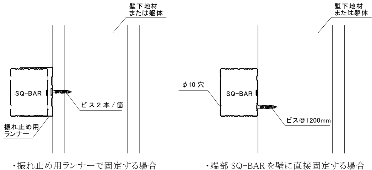
図 2-4-3 短手方向壁際の納まり詳細
