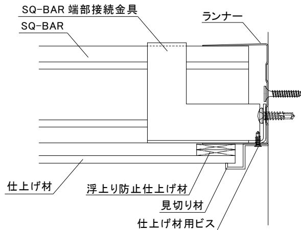
図 3-3-2 見切り材の納まり(廊下長手方向 断面図)
