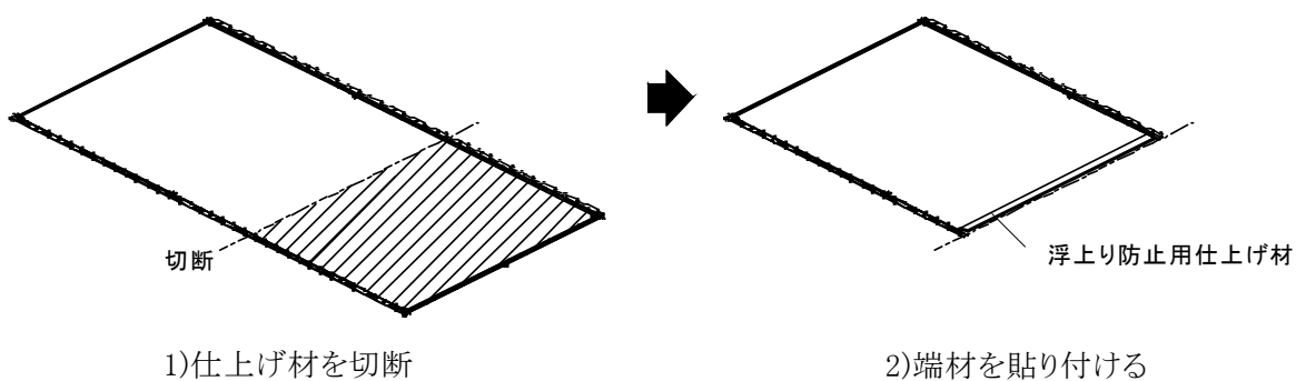
図 3-1-9 壁際に設置する仕上げ材の処理(廊下長手方向)
