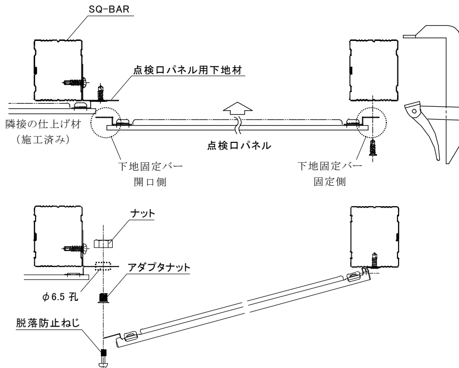
図 3-2-3 点検口パネルの取付け(Y-Y 断面図)
