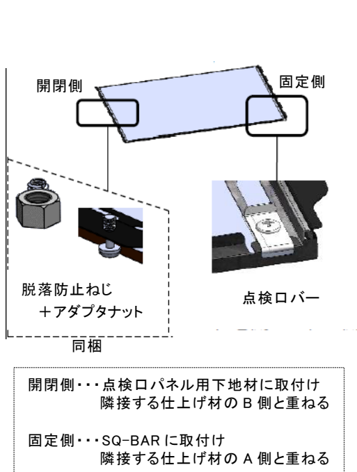
図 3-2-1 エアライト(設備ラインタイプ) 点検口パネル 裏面
