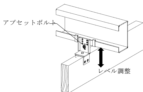
③レベル調整及びアプセットボルトの締込み
