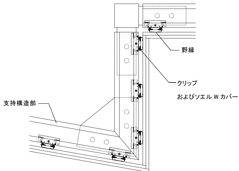
図 3-2-1 (参考例) 勾配、段差部の納まり
