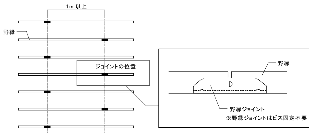
図 2-5-2 野縁の継手
