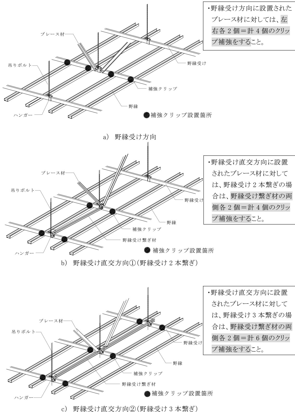
図 2-6-12 補強クリップ設置箇所
