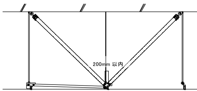
b) 野縁受け直交方向①(野縁受け 2 本繋ぎ)
