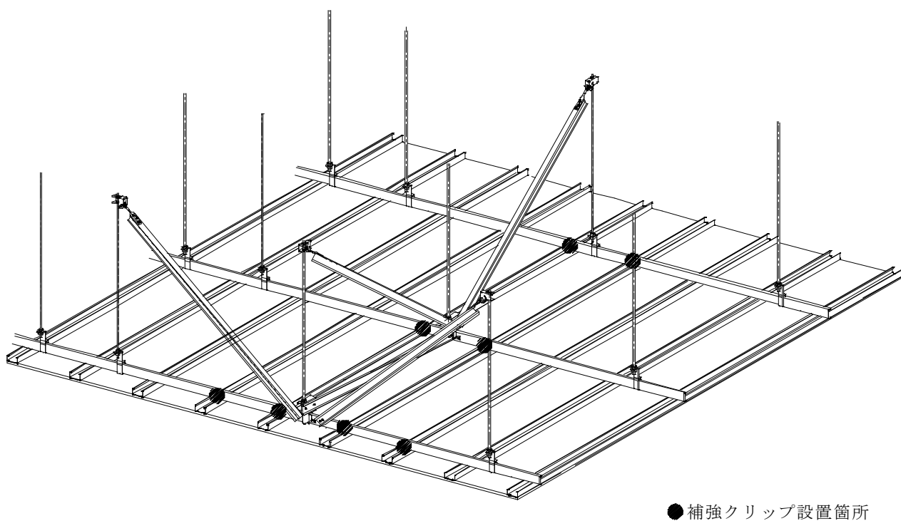
b) 省略配置例
