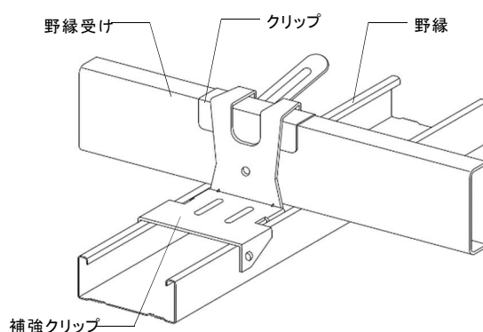
図 2-4-2 壁面と接する周辺部のクリップ
