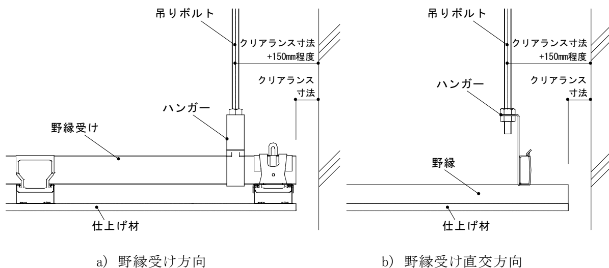
図 2-7-1 (参考例)クリアランスの確認(端部)
