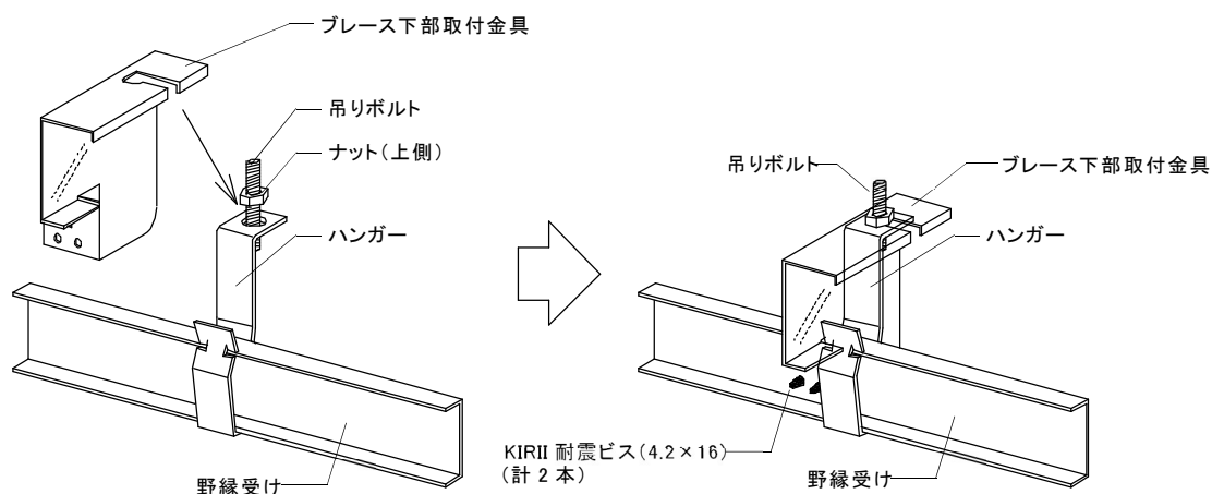
図 2-5-1 ブレース下部取付金具の施工方法
