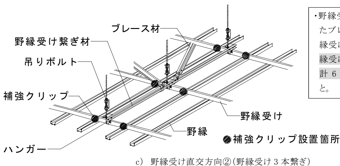
図 2-5-11 補強クリップ設置箇所
