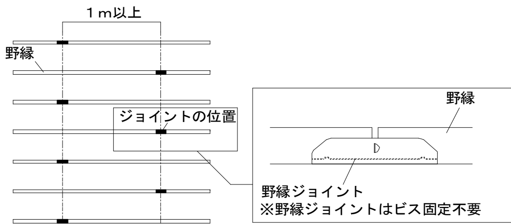
図 2-4-3 野縁の継手
