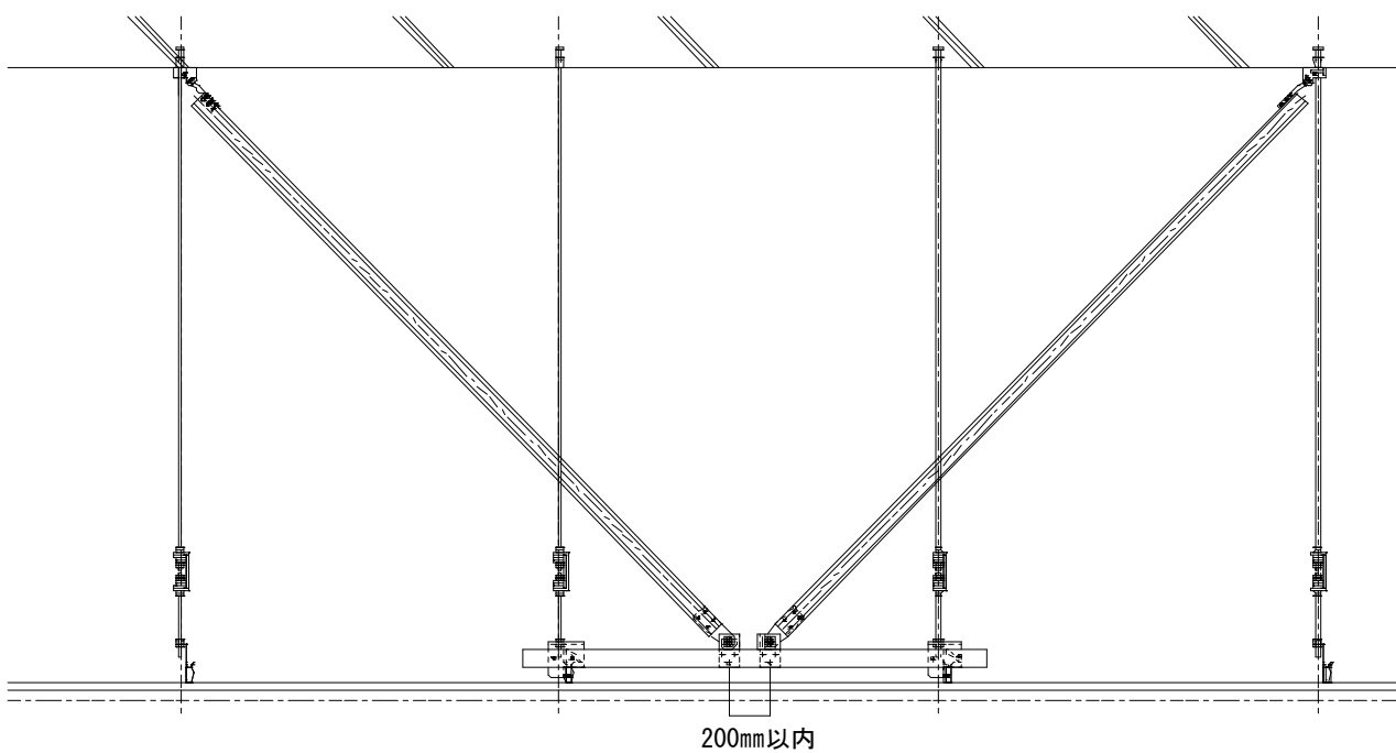
図 2-5-10 ブレース取付け例②
