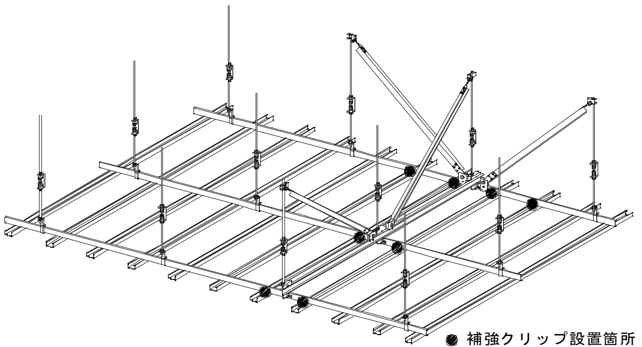
b) 省略配置例
