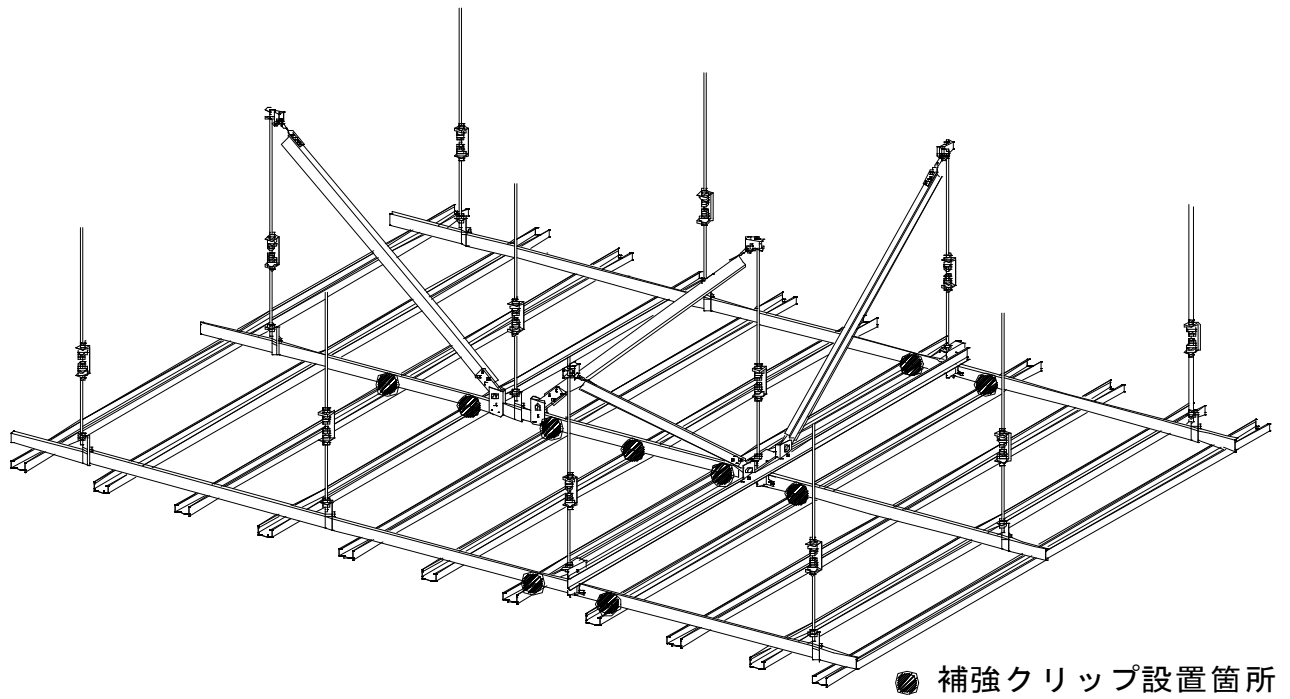
a) 標準配置例
