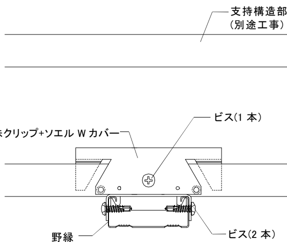
図 2-2-2 ビス固定部詳細
