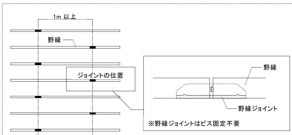
図 2-2-5 野縁の継手
