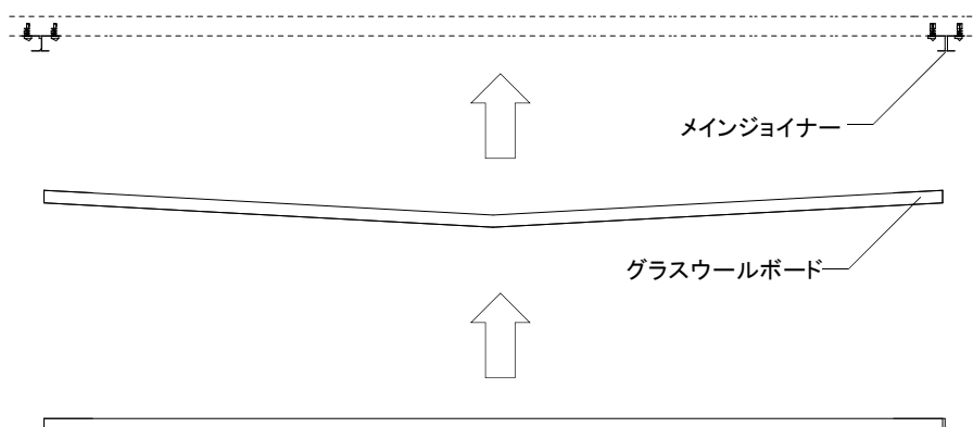
図 2-5-2 グラスウールボードの取付け②
