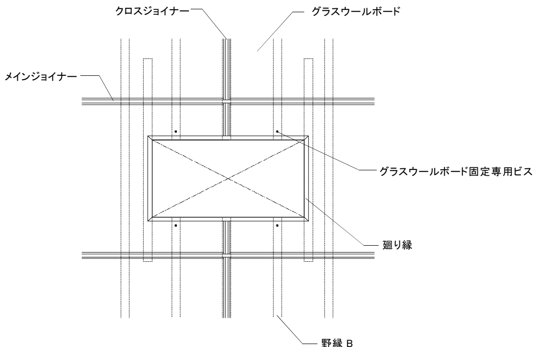
図 3-1-4 ジョイナーが切断される例
