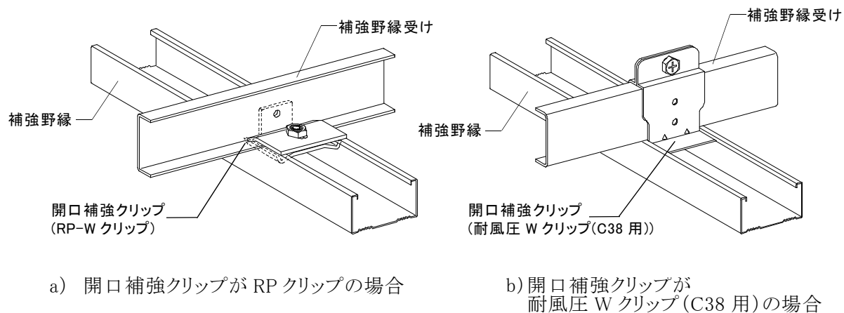
図 3-1-2 開口補強クリップ取付け詳細
