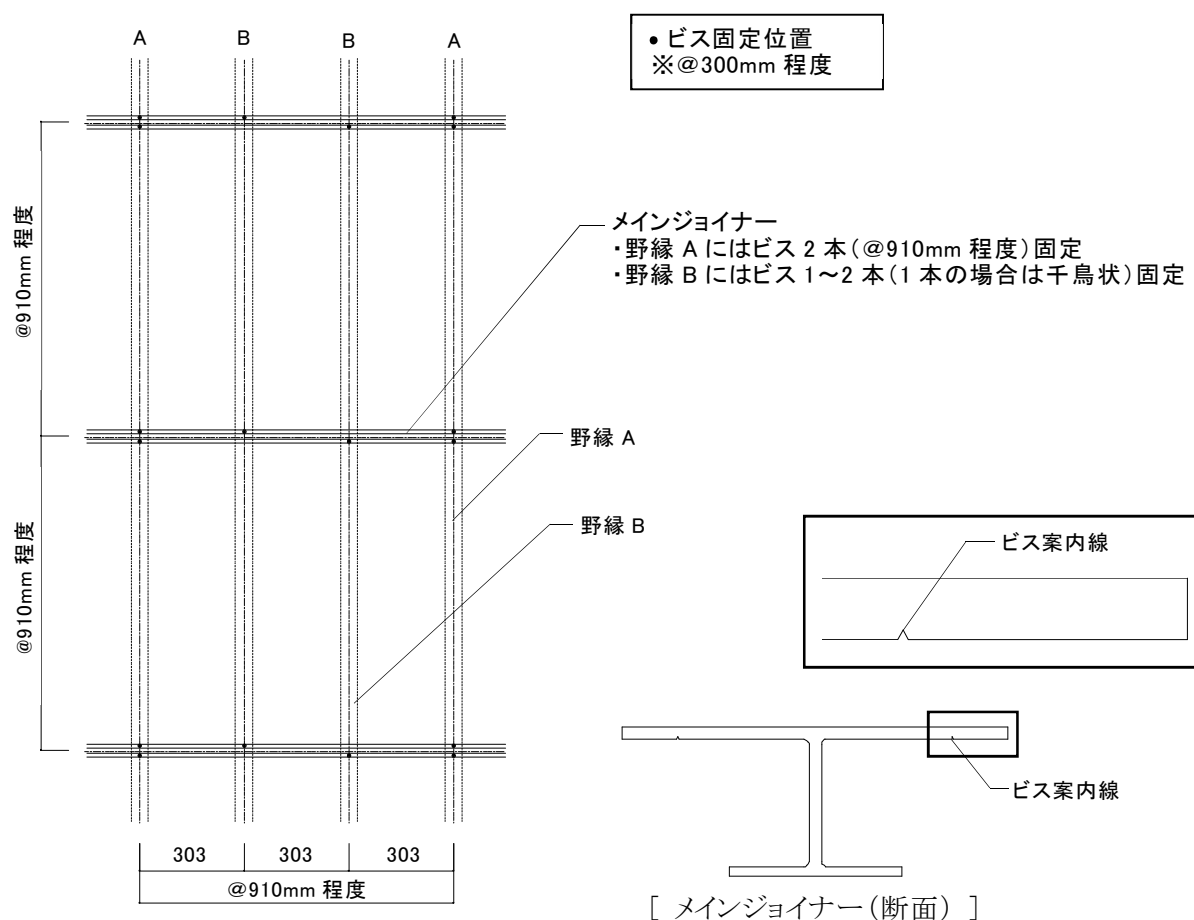
図 2-4-1 メインジョイナーの取付け
