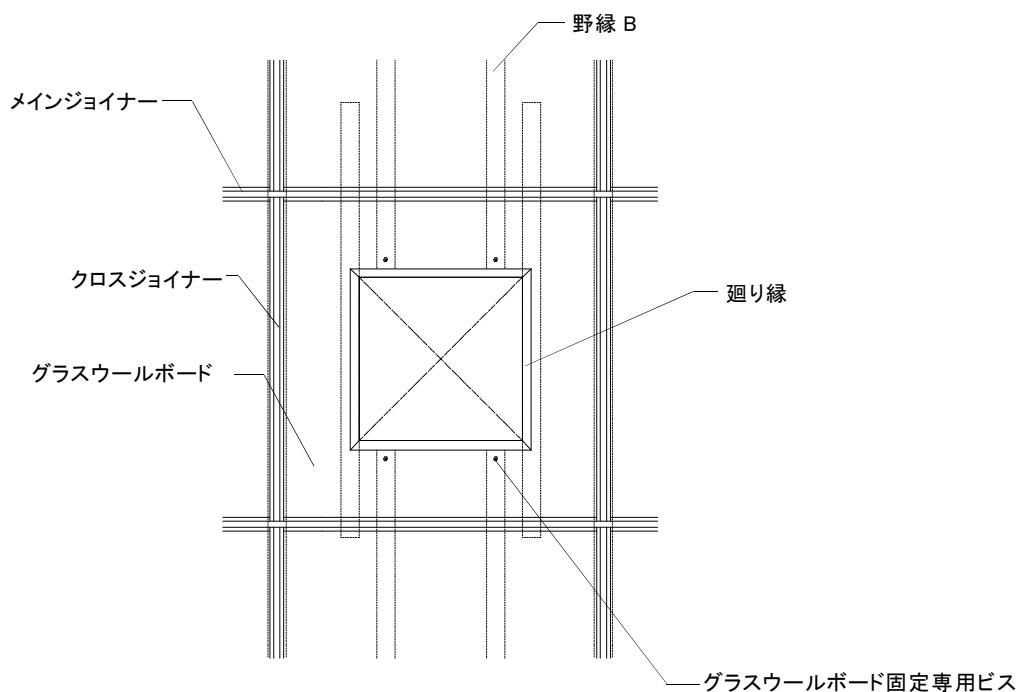
図 3-1-3 ジョイナーが切断されない例
