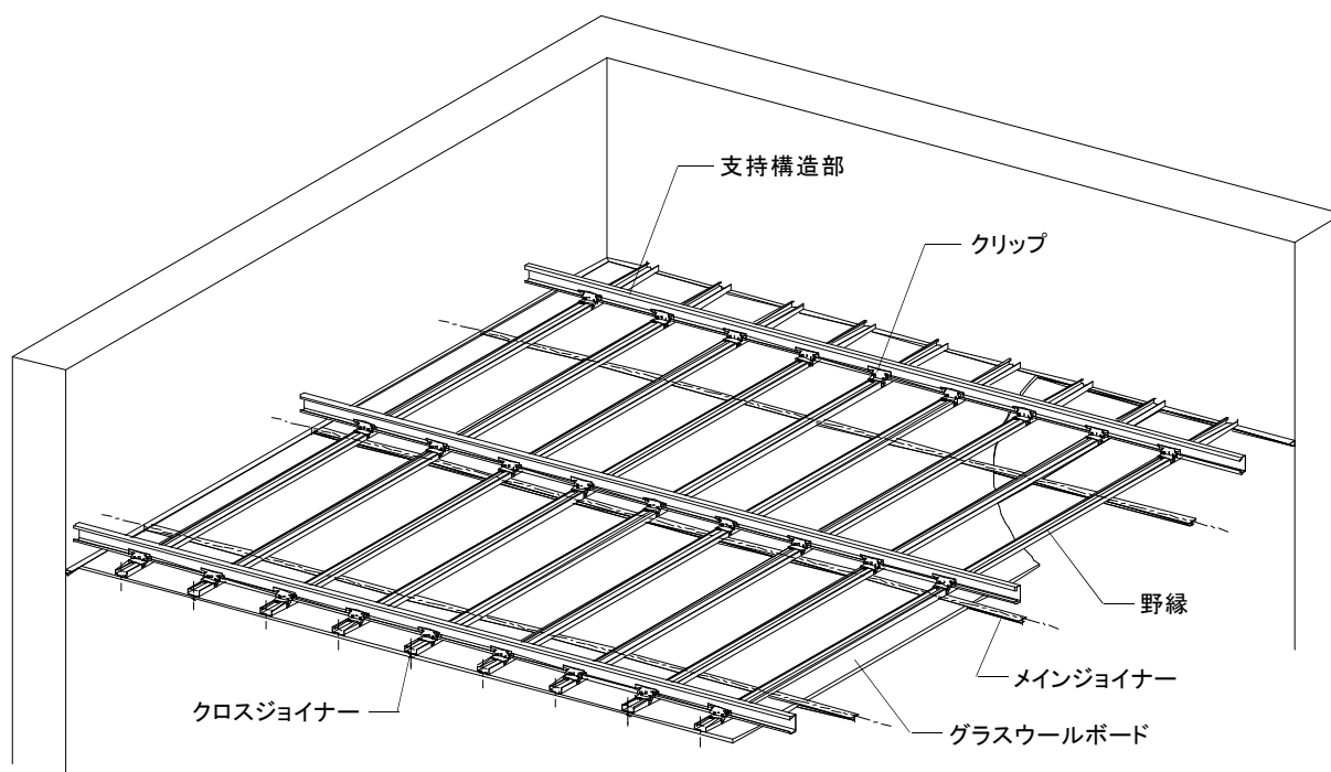
図 1-2-1 (例図) 軽量直張天井(グラスウールボード 12mm 仕様)
