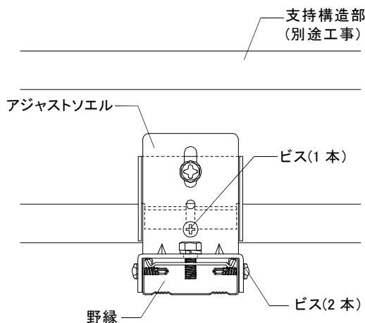
図 2-2-4 ビス固定部詳細
