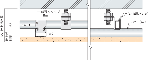
C-19を使用した場合
