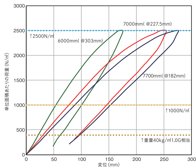
図1 単位面積あたりの荷重-変位曲線
