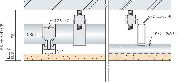
C-38を使用した場合
