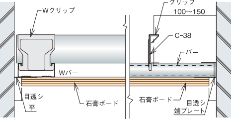
壁納まり（目透板使用の場合）
