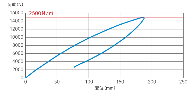
試験 1 荷重-変位曲線 (スタッド間隔303mm)
