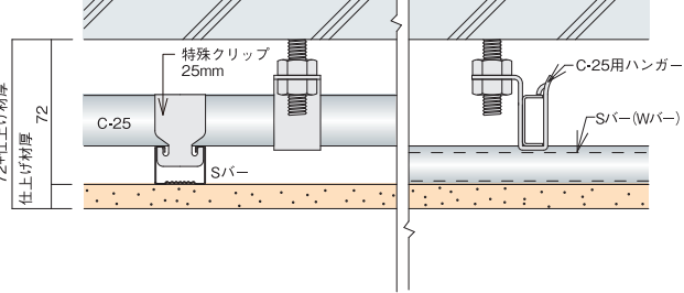
C-25を使用した場合
