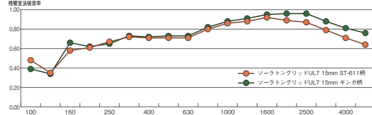
ソーラトングリッドUL7の吸音性能 (15×592×592mm)
