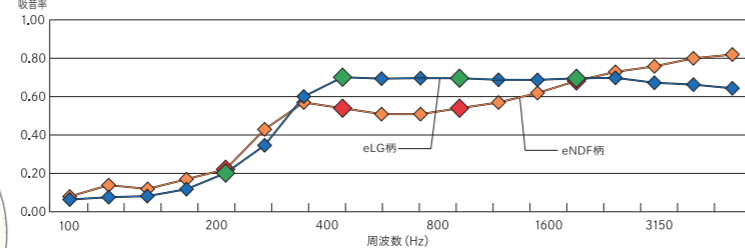
Kロックの吸音性能 (15×593.5×593.5mm)
