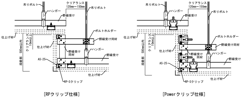
出隅部 AS-25仕様
