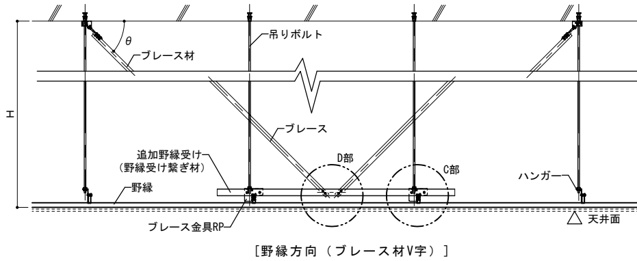
〔野縁方向（ブレース材V字）〕
