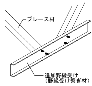
〔D部詳細図〕
