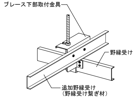
〔C部詳細図〕
