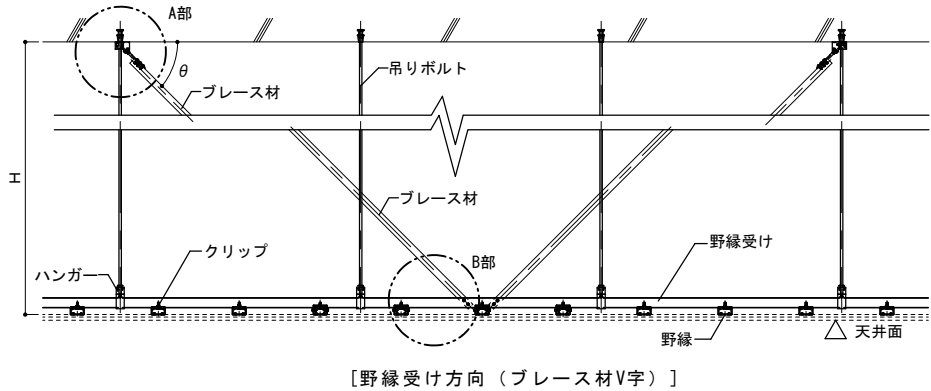
〔野縁受け方向（ブレース材V字）〕
