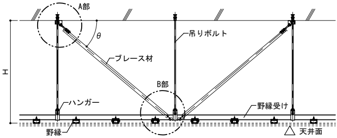
〔野縁方向（ブレース材V字）〕
