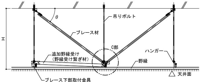
〔野縁受け方向（ブレース材V字）〕
