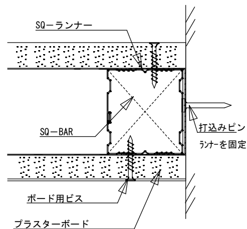
A-A' 断面図
