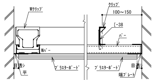
壁納まり（目地板使用の場合）
