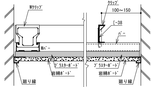
壁納まり（廻り縁使用の場合）
