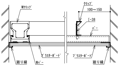
壁納まり（廻り縁使用の場合）
