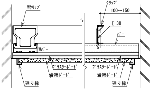
壁納まり（廻り縁使用の場合）
