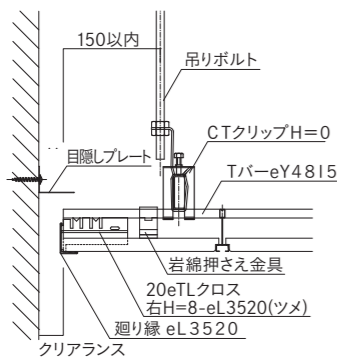
■壁際との納まり例 3
