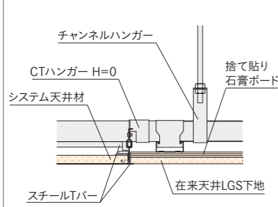
■在来天井との納まり
