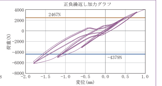
斜め部材 AS-25 (25×19×5×1.0)
