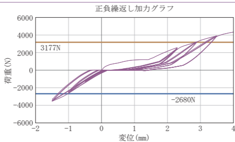
野縁受け CC-19
