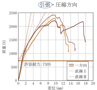
一方向加力グラフ
