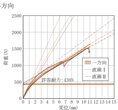
野縁受け方向一方向加力グラフ
