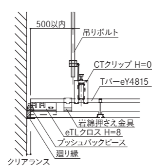
■防煙垂壁の納まり例
