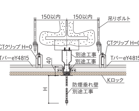
■防煙垂壁の納まり例
