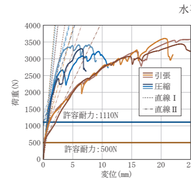
野縁方向一方向加力グラフ
