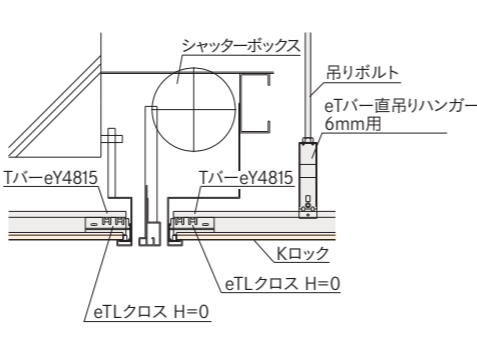
■シャッターボックスの納まり
