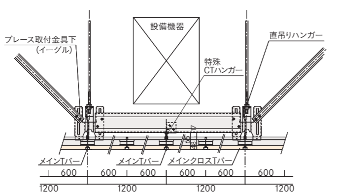
■設備機器周りの補強例
