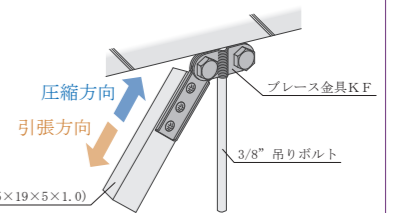
斜め部材 AS-25 (25×19×5×1.0)
