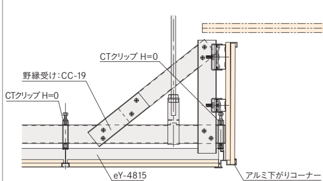
■下り天井の納まり ②
