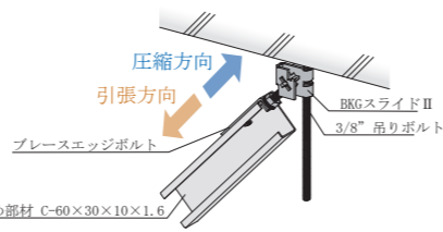
斜め部材 C-60×30×10×1.6
