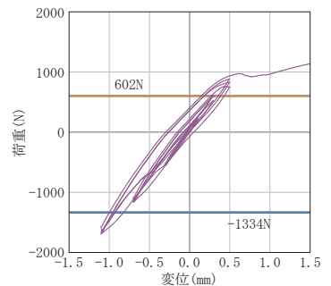
野縁方向繰返し加力グラフ
