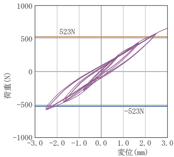
野縁受け方向繰返し加力グラフ
