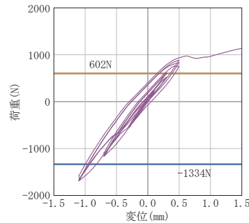
野縁方向繰返し加力グラフ
